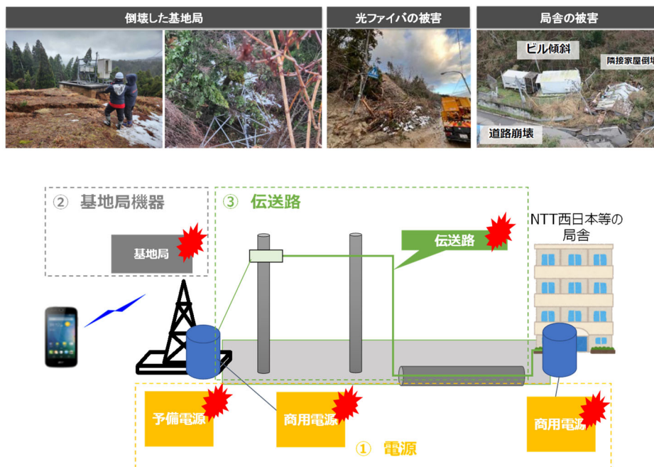
図4 携帯電話ネットワークの支障の原因
