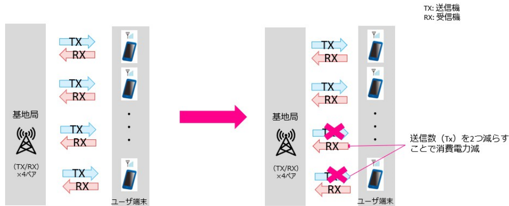
図 13 楽天モバイルの取組例（基地局の省電力運用）
