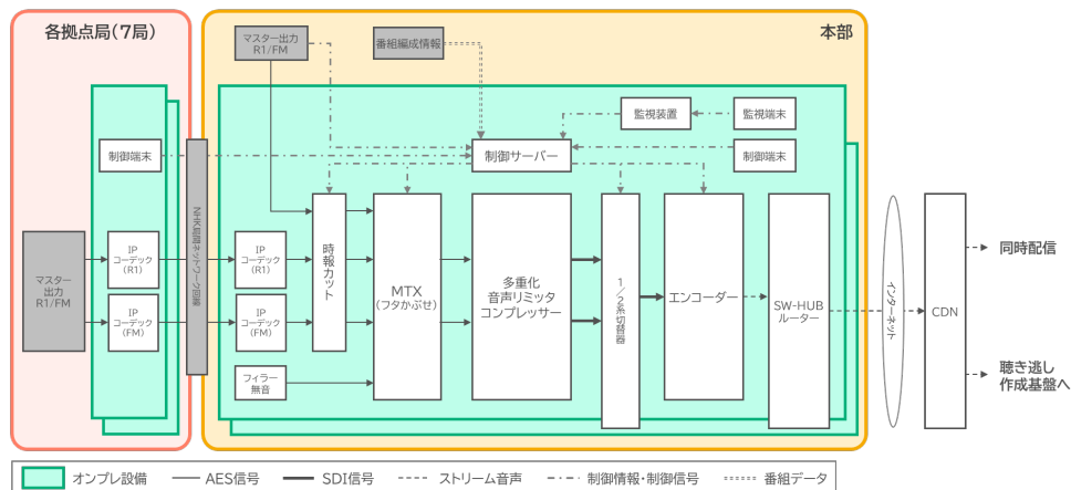
国内ラジオ同時配信系統(オンプレ)
