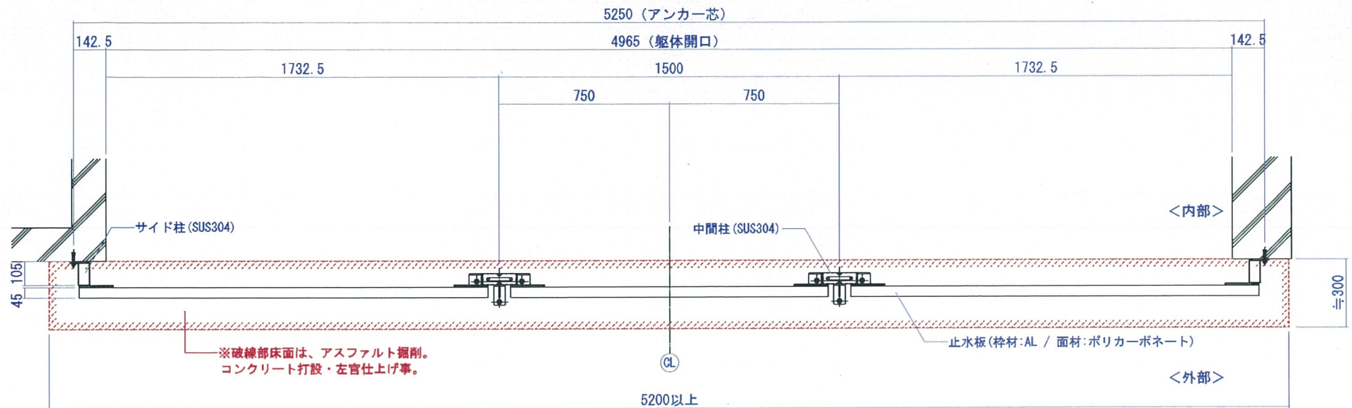
平面図
