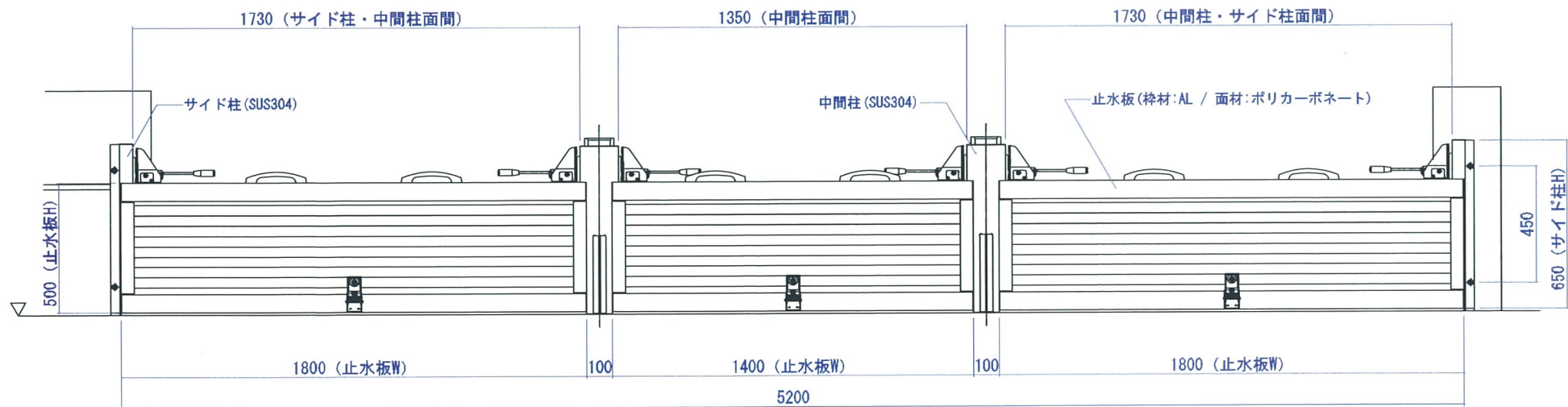
外観立面図
