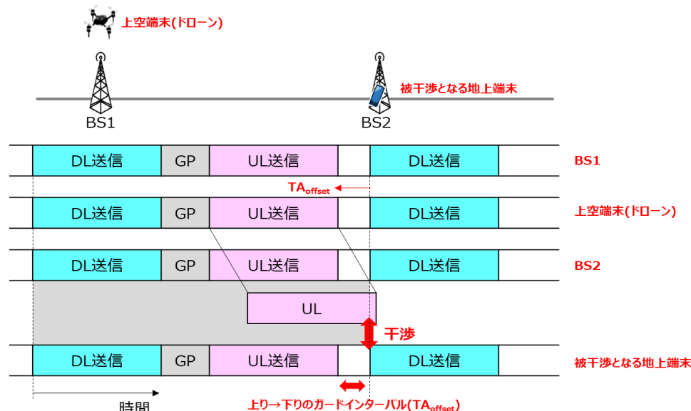
過去の検討※における遠方捕捉問題の説明
