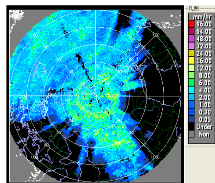
気象レーダーの降雨観測(画面例)
