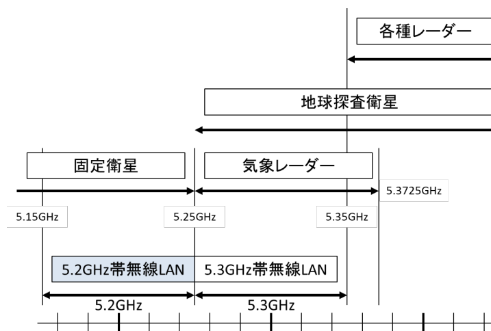
図 4-1-1 5.2GHz帯の使用状況
