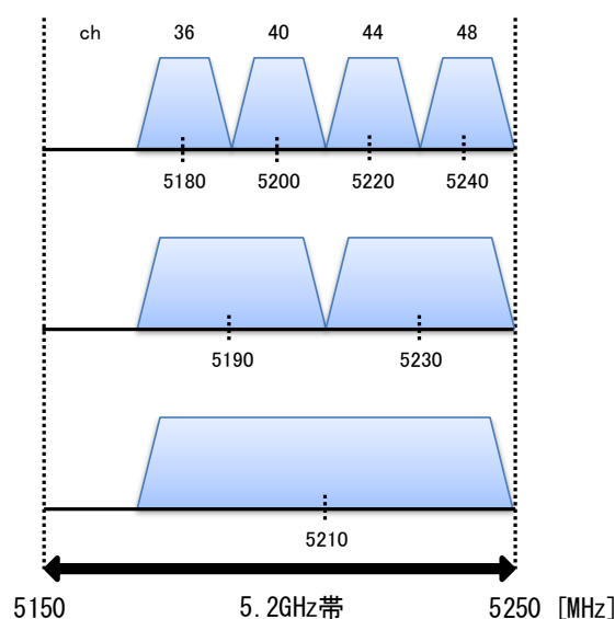
図 5-2-1 5. 2GHz 帯無線 LAN の上空利用に係る周波数チャネル配置図
