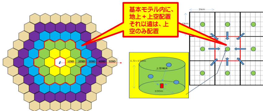
遠方捕捉問題の検討モデル (左: 2.5GHz帯、Sub6帯の場合、右: mmW帯の場合)
