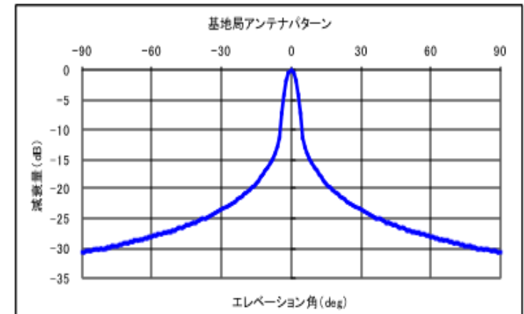
図2 BWA基地局のアンテナパターン
