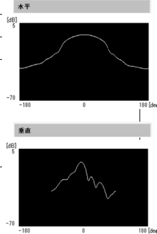
図1 HPUE(PC1)アンテナパターン
