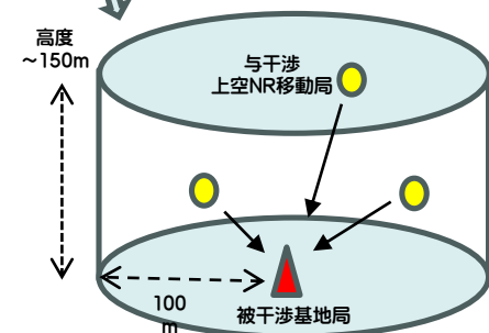
図2 mmW帯でモンテカルロシミュレーションにより携帯電話等基地局への影響を評価する場合の検討モデル
