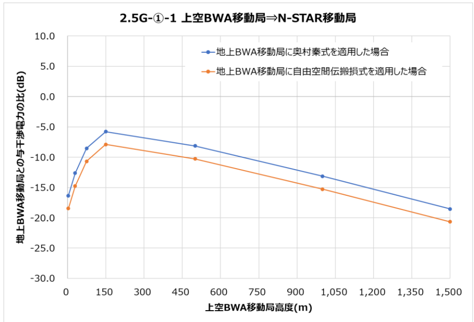
2.5G-①-1 上空BWA移動局⇒N-STAR移動局
