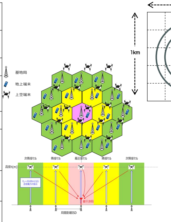
図1 BWA帯、Sub6帯でモンテカルロシミュレーションにより携帯電話等基地局への影響を評価する場合の検討モデル
