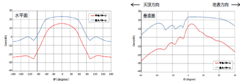
図3 mmW帯NR基地局アンテナパターン(左:水平、右:垂直)
