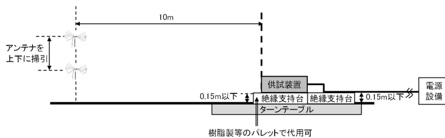
別図第十二号 三〇MHz を超え一、〇〇〇MHz 以下の利用周波数による発射及び不要発射による電界強度の測定（搬送ロボット用非接触電力伝送装置）
