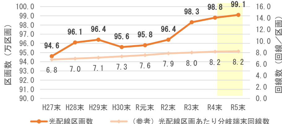
光配線区画の状況（NTT西日本）
