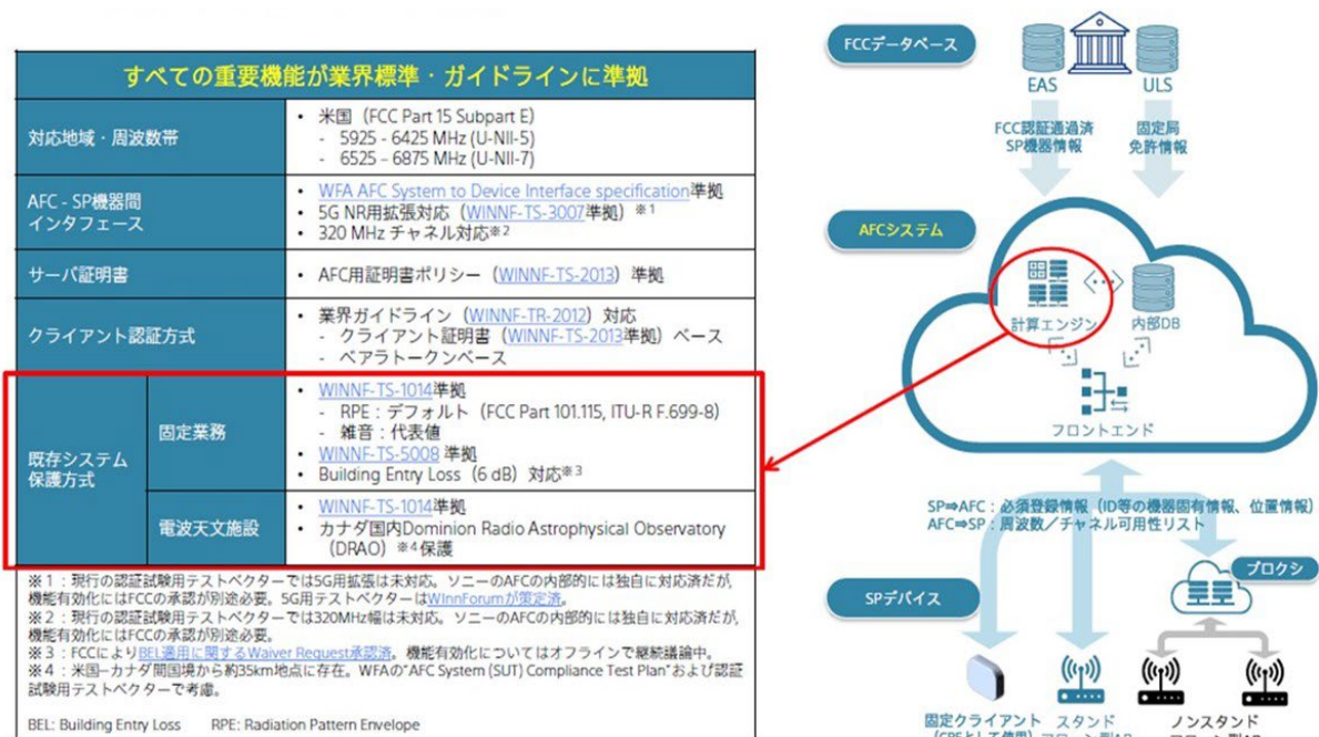
図 参-1 ソニー社 AFC システム基本仕様
