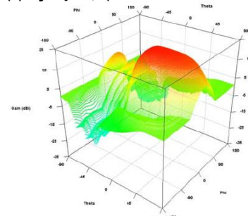
5G基地局の空中線指向特性
