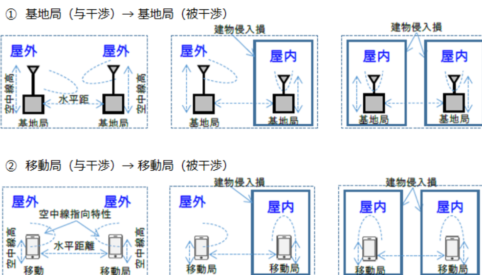
図 2. 2-19 40GHz 帯 5G システム相互間の共用検討（同一周波数：非同期運用）＜シナリオ 1-b＞
