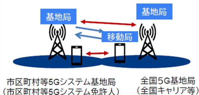
図 2. 2-20 40GHz 帯 5G システム相互間の共用検討（隣接周波数：非同期運用）＜シナリオ 2＞
