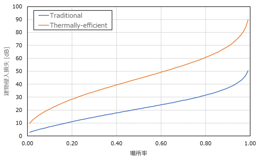
図 2. 2－17 40GHz 帯 建物侵入損
