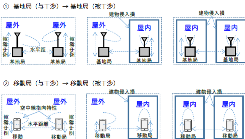
図 2. 2-21 40GHz 5G システム相互間の共用検討（同一周波数：非同期運用）＜シナリオ 2＞
