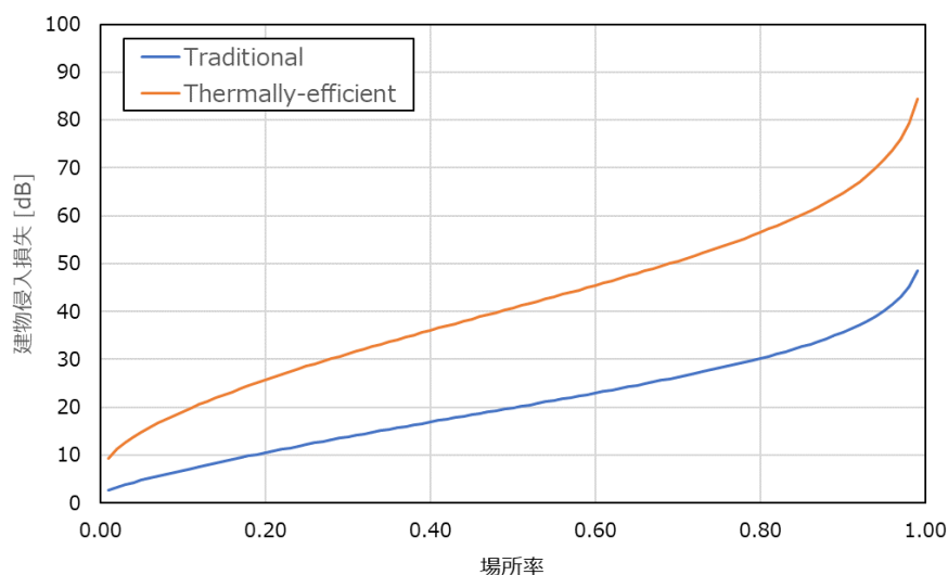
図 2. 1－17 26GHz 帯 建物侵入損
