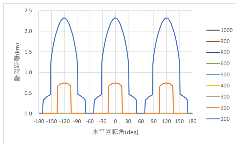
図 2. 1－14 シナリオ 2-b の検討結果
