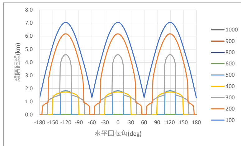
図 2. 1-1-2 シナリオ 1-a の検討結果
