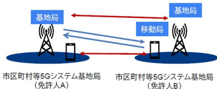
図 2. 2-18 40GHz 帯 5G システム相互間の共用検討の概要（同一周波数：非同期運用）＜シナリオ 1-b＞
