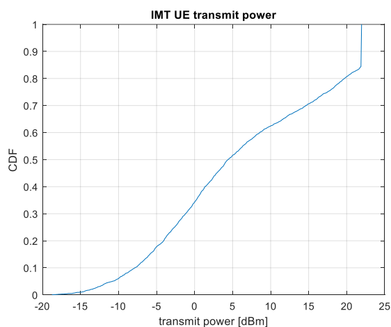
図 2. 2-23 移動局の送信電力分布
