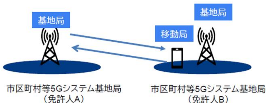
図 2. 2-15 40GHz 帯 5G システム相互間の共用検討の概要（同一周波数：同期運用）＜シナリオ 1-a＞
