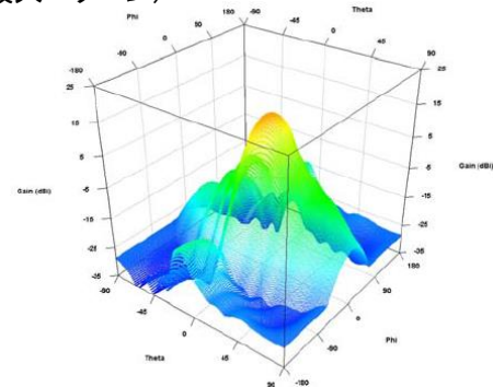
図 2. 1-3 26GHz 帯 5G 基地局の空中線指向性
