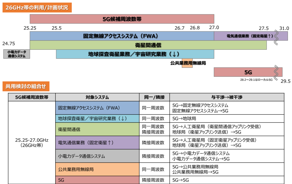
図 2. 1－1 共用検討対象となる無線システム (26GHz 帯)
