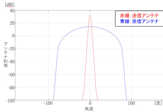
アンテナ放射パターン（ホーム画像伝送システム・水平）
