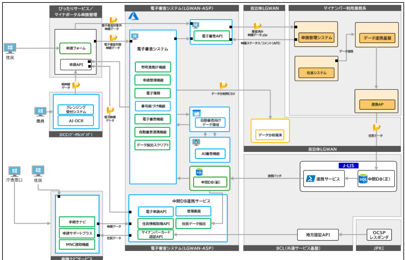
図表 7-4 システム構成概略図
