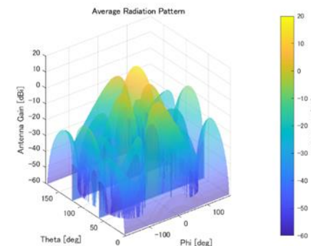
5G移動局の空中線指向特性
