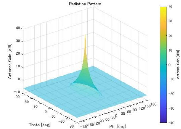
40GHz帯 FPUシステムの空中線指向特性
