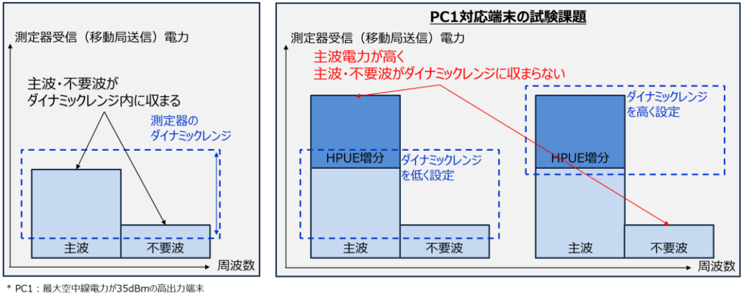
図 1. 3－8 測定器のダイナミックレンジ
