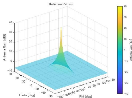
図 2. 2-8 38GHz 帯 FWA の空中線指向性
