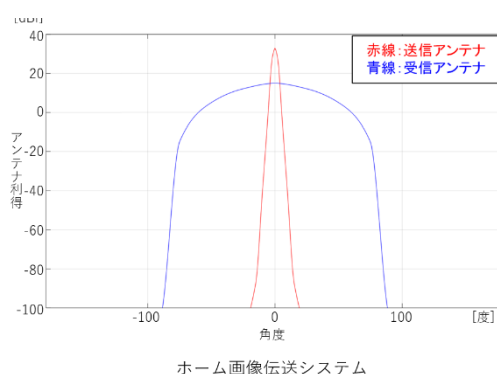
図 2. 2-15 検討に用いたアンテナの放射パターン（水平）
