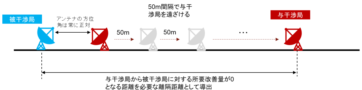
図 2. 1－5 1 対 1 対向シミュレーションの概念図
