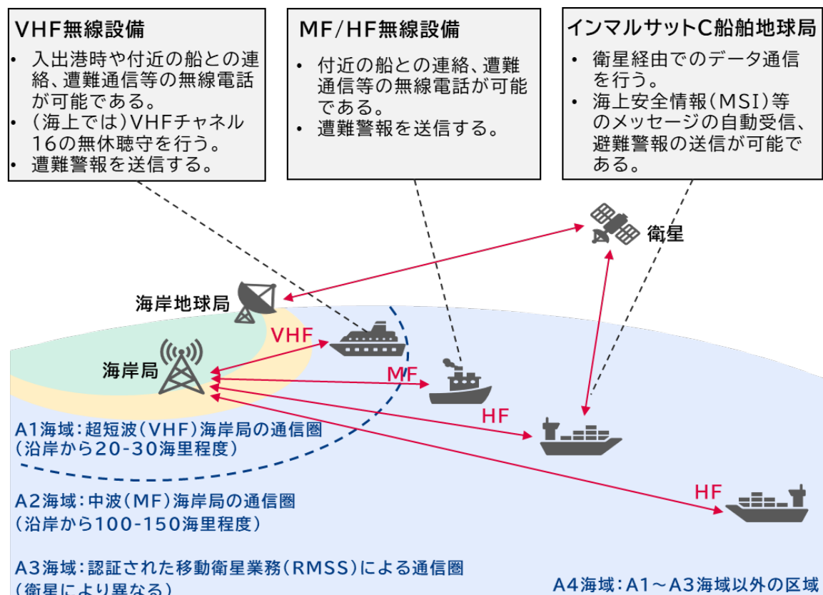
図 2-1 主な GMDSS 船舶用無線機器の利用イメージ①
