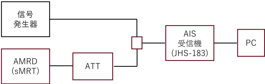
図 4-11 Group A 干渉試験の測定系
