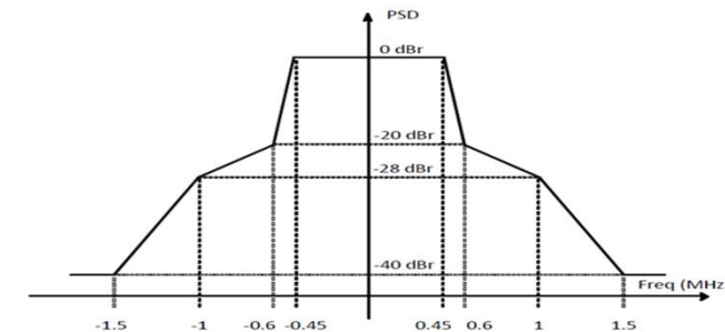
図4 送信スペクトラムマスク特性
