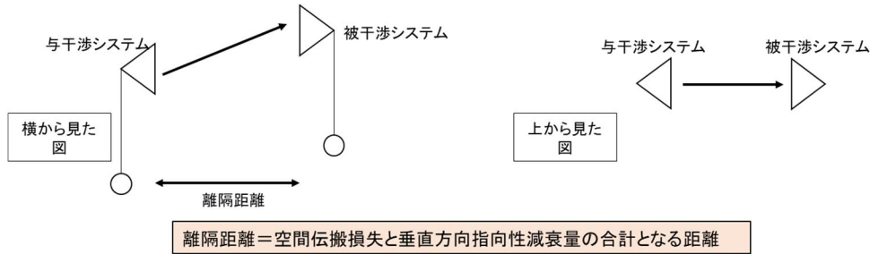
図 3.1-4 1対1対向モデル（アンテナ高低差等を考慮したモデル）
