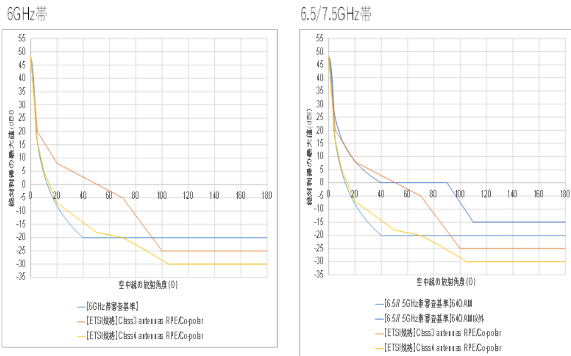
図 2-1 現行審査基準及び ETSI 規格空中線特性
