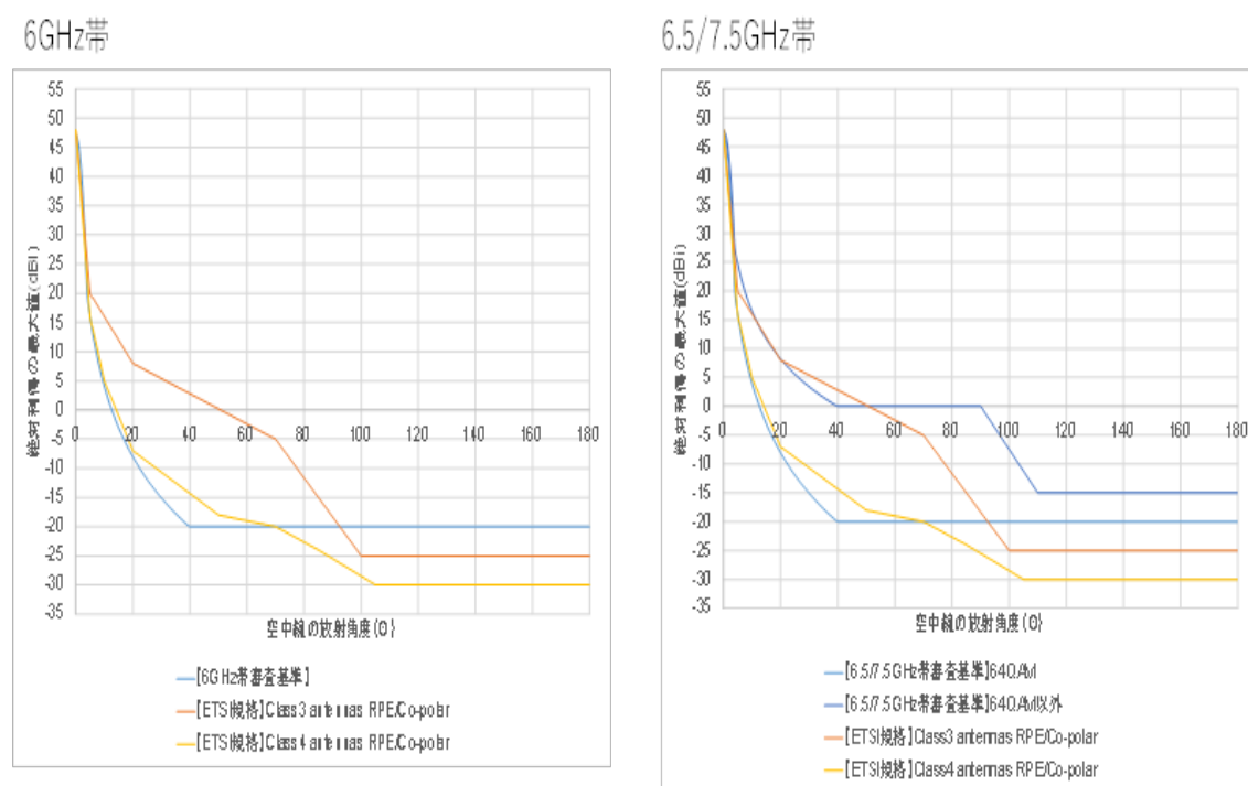
図 2-4 現行審査基準及び ETSI 規格空中線特性
