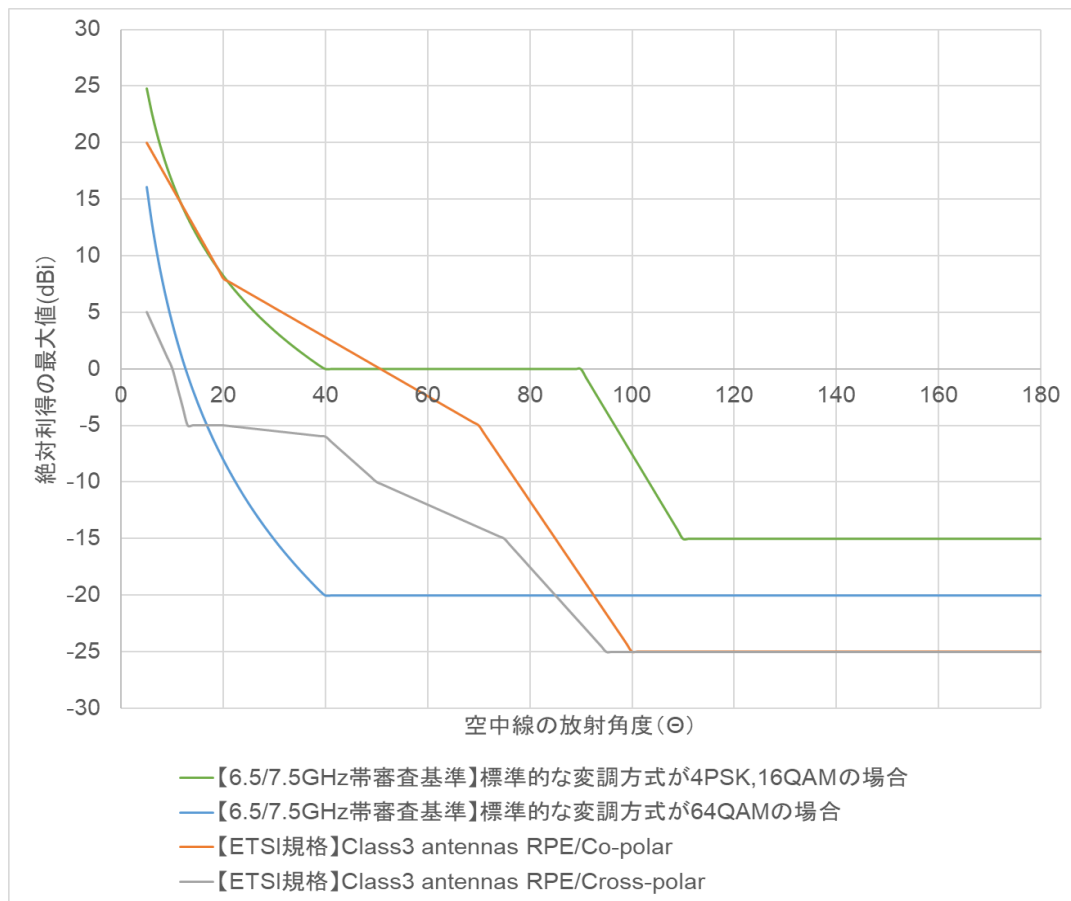
図 1-18 ETSI 規格と 6.5/7.5GHz 帯審査基準における、標準受信空中線特性の比較 出所)各種資料を基に、三菱総合研究所作成
