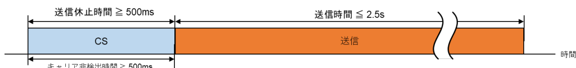
図参 5.2.1 WPT キャリアセンスの動作
