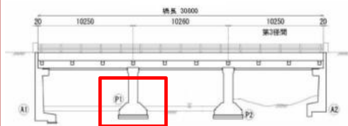
橋梁側面図
