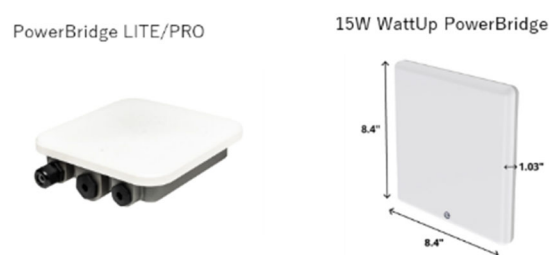
図 1.2.8 Energous 社の WPT 送電装置※6
