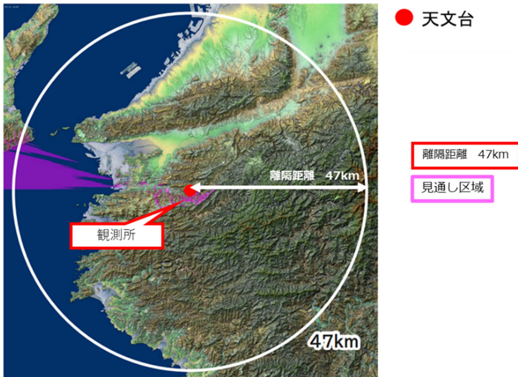
図 3. 3. 3 和歌山大学みさと天文台における 空間伝送型ワイヤレス電力伝送システムの制限区域
