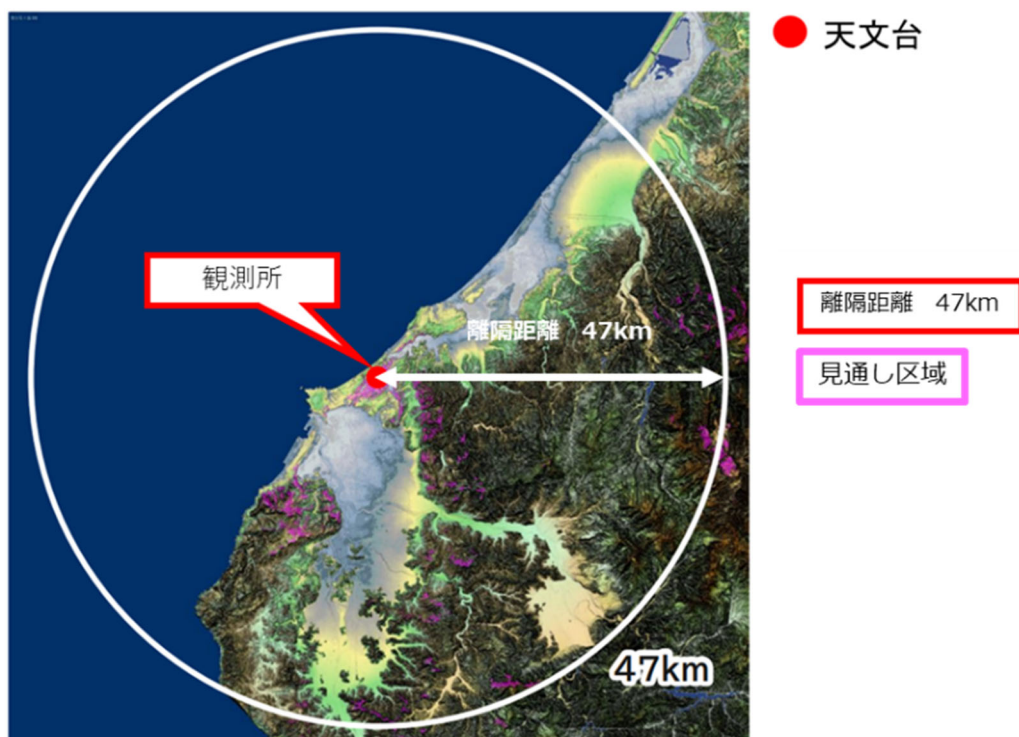
図 3.3.6 福井工業大学あわら宇宙センターにおける 空間伝送型ワイヤレス電力伝送システムの制限区域
