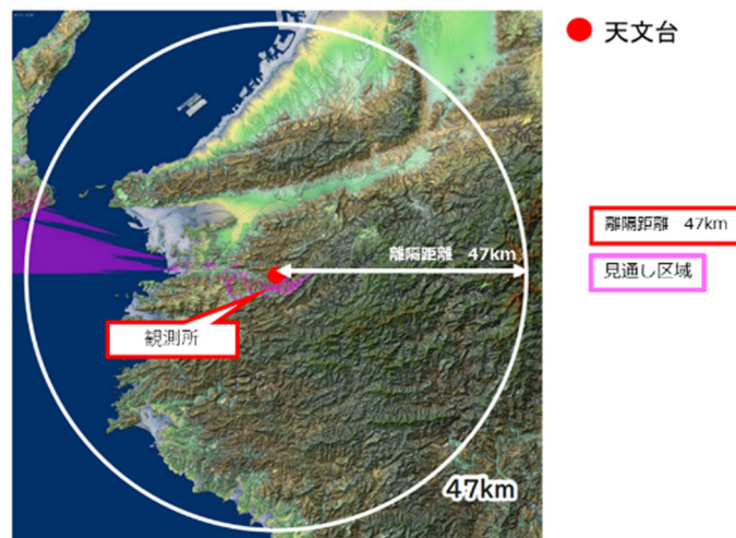
図参 4. 2. 3 和歌山大学みさと天文台における 空間伝送型ワイヤレス電力伝送システムの制限区域
