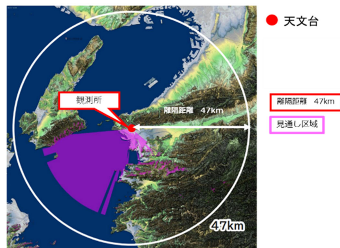
図参 4. 2. 4 和歌山大学和歌山大 12m における 空間伝送型ワイヤレス電力伝送システムの制限区域
