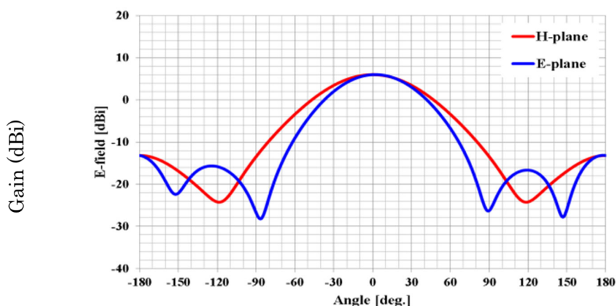
図 3.2.1 920MHz 帯 空中線指向特性
