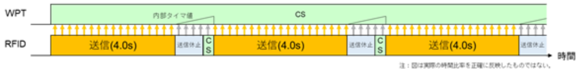
(b) 4 秒間送信の RFID とのキャリアセンス動作例
