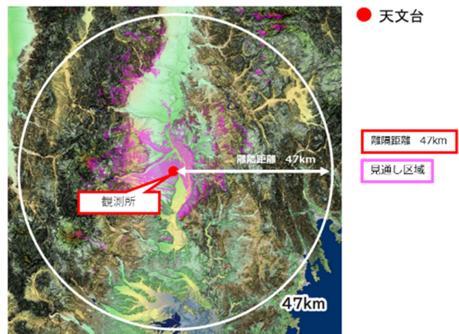
図参 4. 2. 6 福井工業大学あわら宇宙センターにおける空間伝送型ワイヤレス電力伝送システムの制限区域
