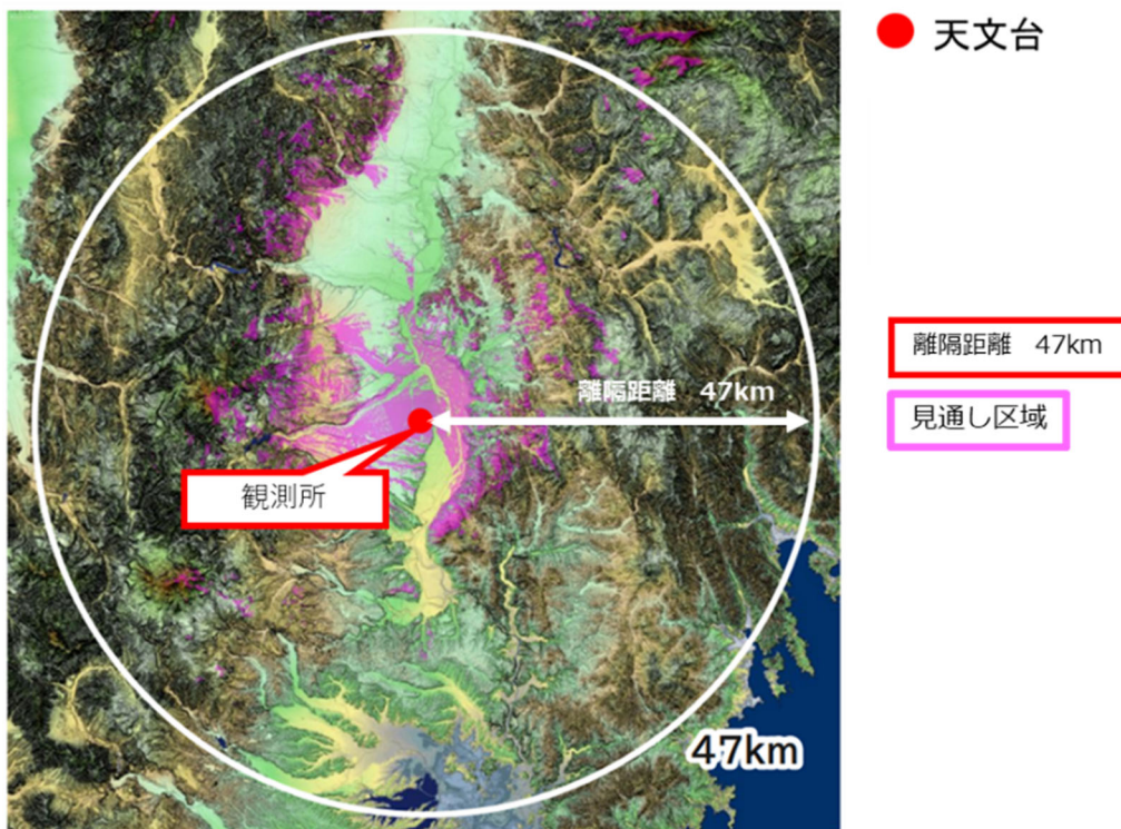
図 3.3.7 国立天文台水沢 VLBI 観測所における 空間伝送型ワイヤレス電力伝送システムの制限区域
