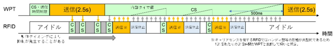
(a) 短時間動作 RFID とのキャリアセンス動作例
