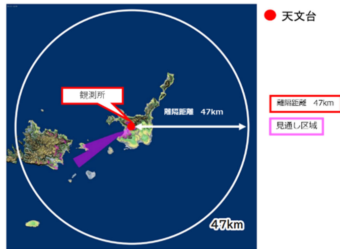
図参 4.2.8 国立天文台 VERA 石垣島観測所における 空間伝送型ワイヤレス電力伝送システムの制限区域
