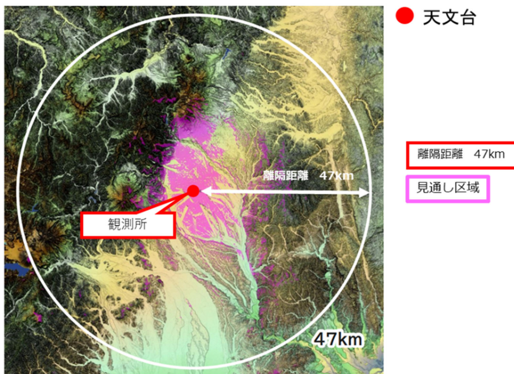
図 3.3.5 自由学園那須農場電波観測所における 空間伝送型ワイヤレス電力伝送システムの制限区域
