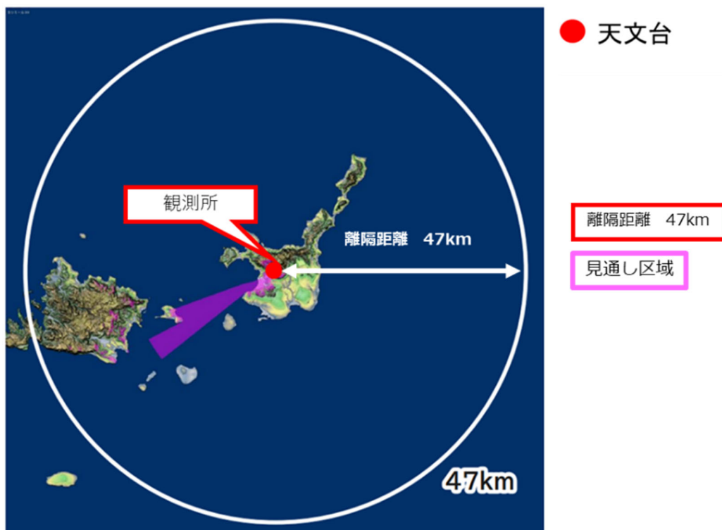
図 3.3.8 国立天文台 VERA 石垣島観測所における 空間伝送型ワイヤレス電力伝送システムの制限区域
