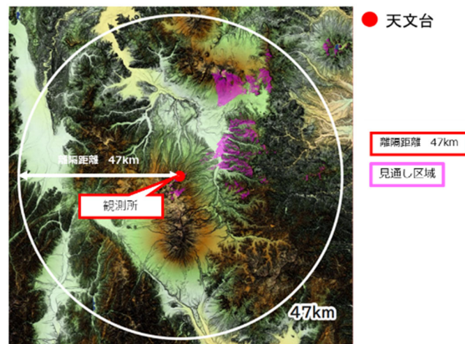
図参 4. 2. 2 JAXA 白田宇宙空間観測所における 空間伝送型ワイヤレス電力伝送システムの制限区域
