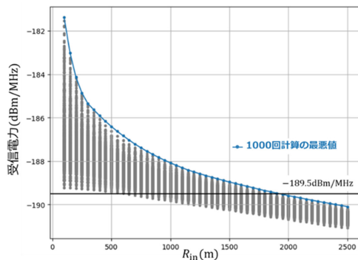
図 3.3.15 モンテカルロシミュレーション結果
