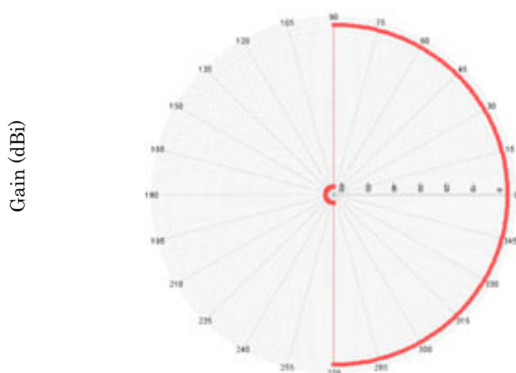
図 3.2.2 920MHz 帯 特定小電力型 WPT システムの空中線指向特性
