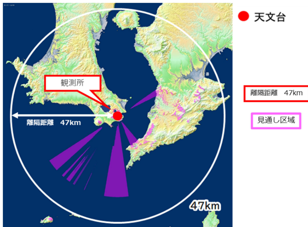
図 3. 3. 9 NICT 山川局における 空間伝送型ワイヤレス電力伝送システムの制限区域
