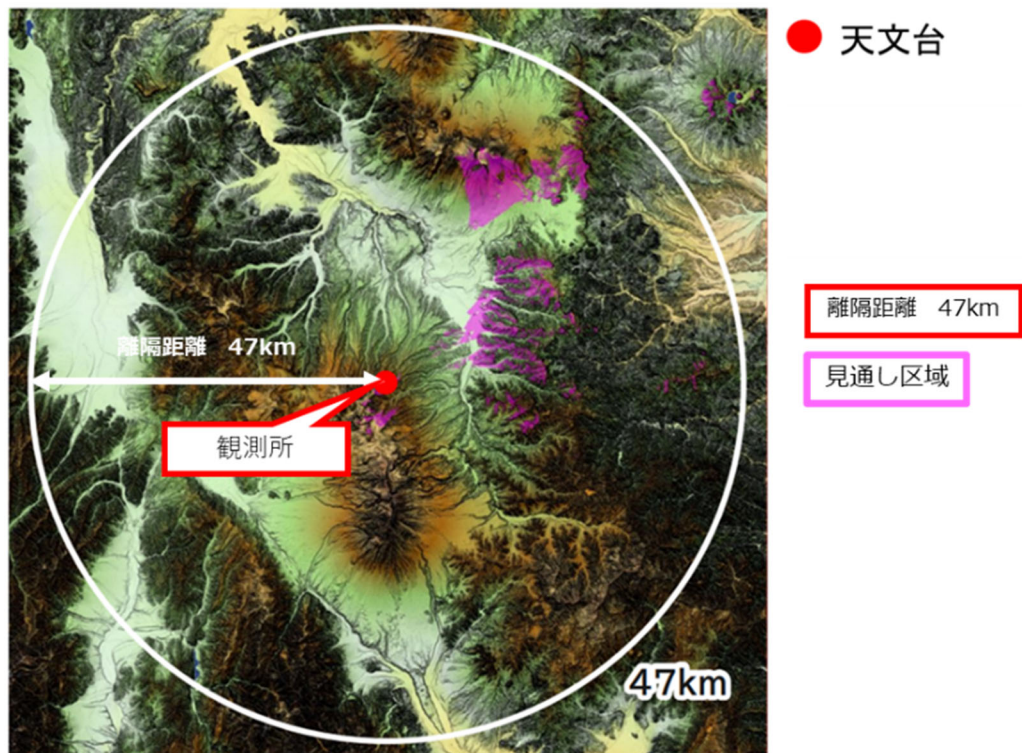
図 3.3.2 JAXA 白田宇宙空間観測所における 空間伝送型ワイヤレス電力伝送システムの制限区域
