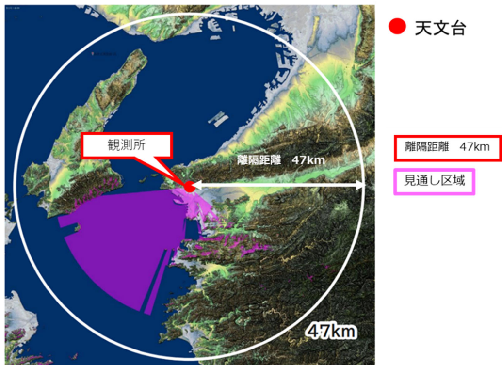
図 3. 3. 4 和歌山大学和歌山大 12m における 空間伝送型ワイヤレス電力伝送システムの制限区域
