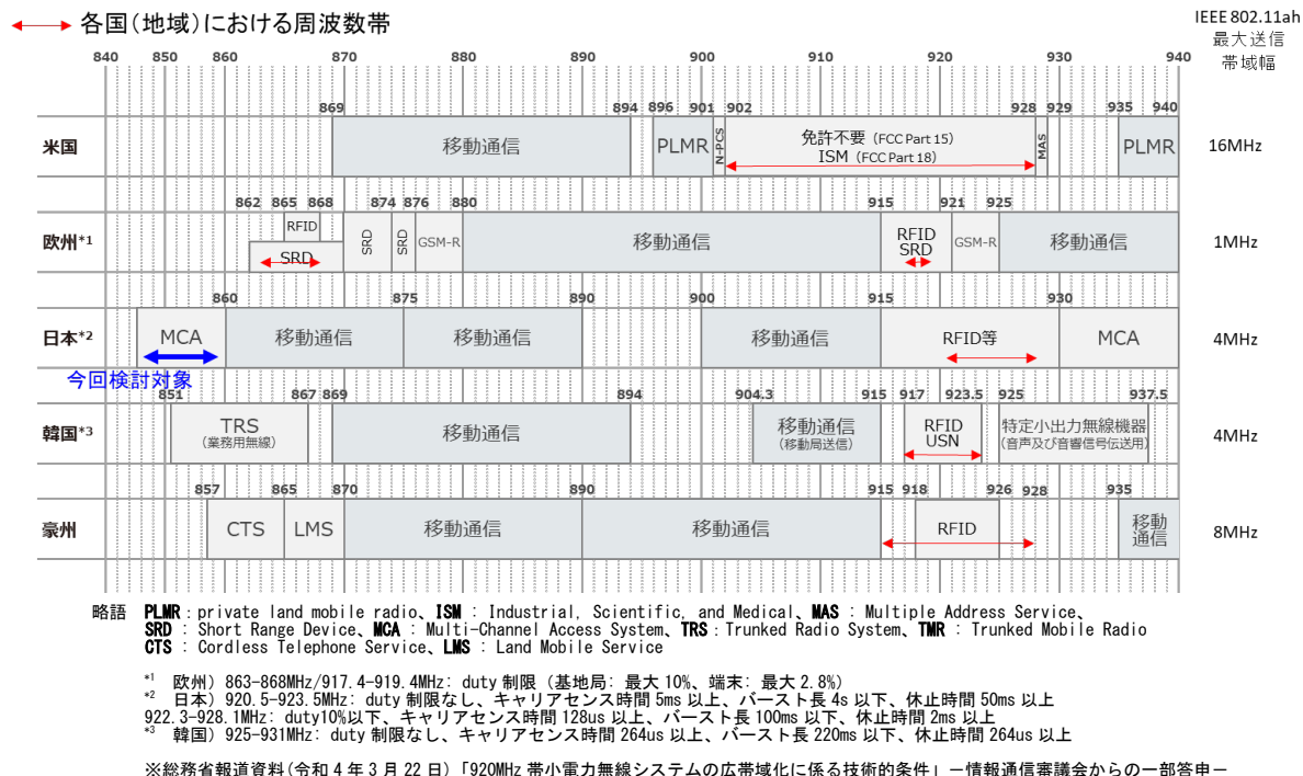
図 2.2-6 802.11ah システムの各国のプランバンド
