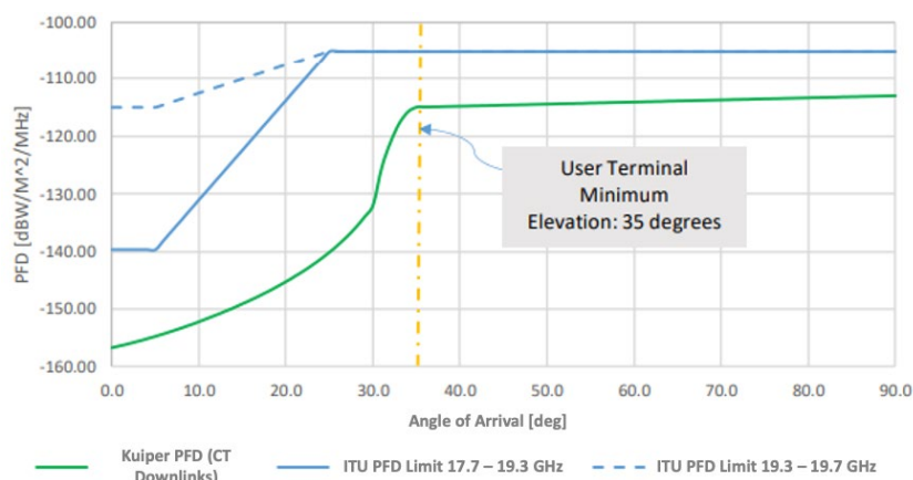
図 4. 1. 2-1 Ka 帯非静止衛星通信システム（600km）（衛星局）（地球局対向）の PFD について
