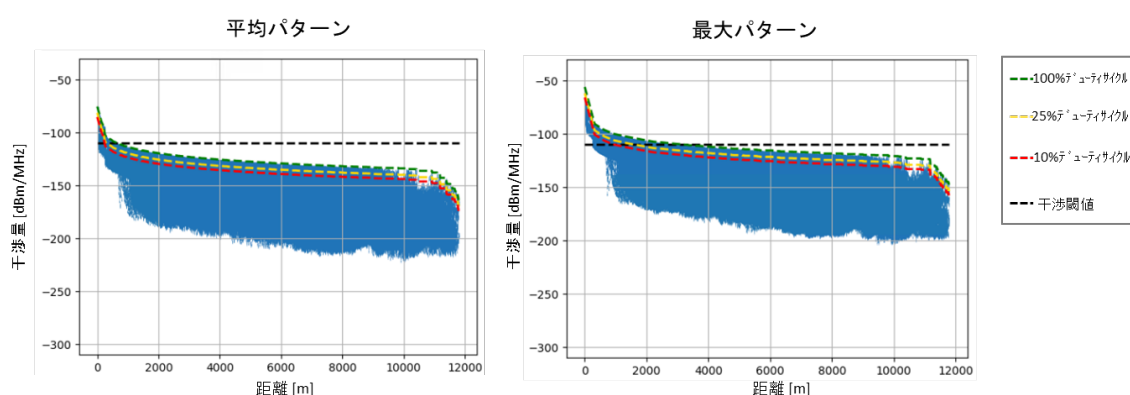
図4. 2. 2－4 干渉検討結果（屋外設置、アンテナ高 10m、近郊クラッタ考慮）
