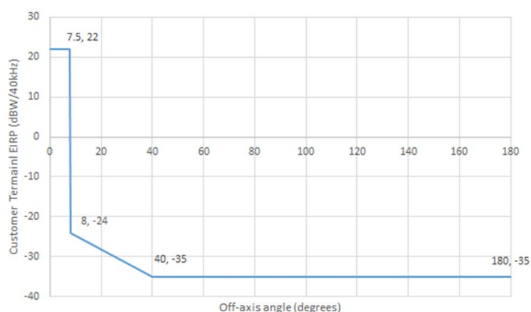
図 2. 3. 1-1 Ka 帯非静止衛星通信システム（地球局）の EIRP 密度（軸外）
