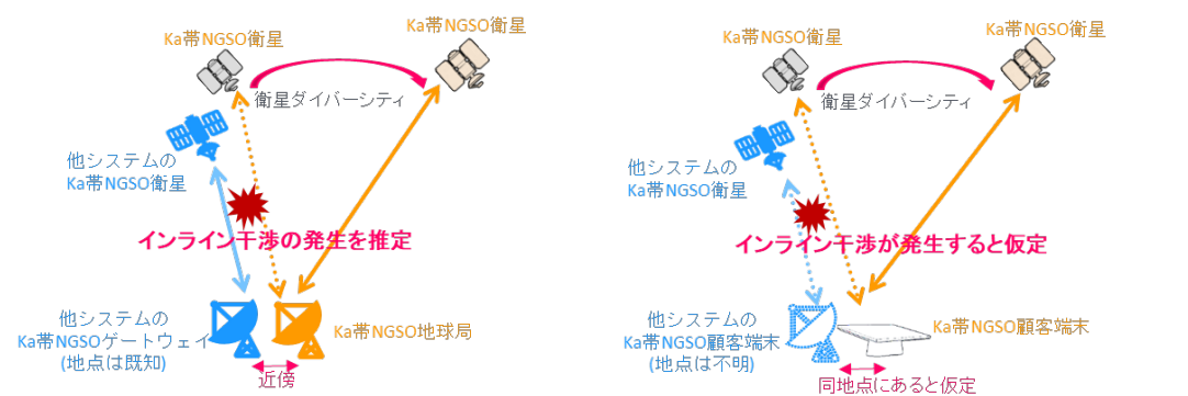
図 1. 2. 3-2 エフェメリスデータを用いたインライン干渉回避策
