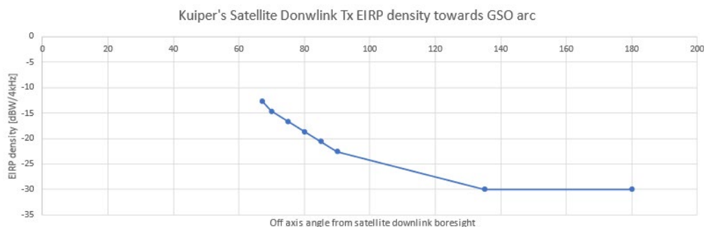
図2. 3. 2-3 Ka 帯非静止衛星通信システム（衛星局）の EIRP 密度（参考）
