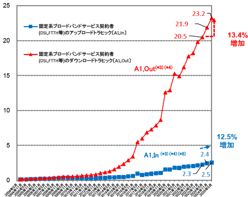
(Tbps) 固定系 broadband サービス契約者のトラフィック[A1]の推移
