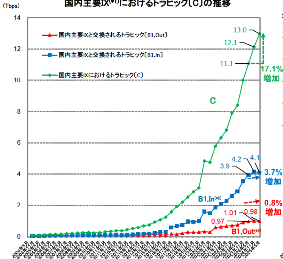
国内主要IX(*1)と交換されるトラフィック[B1] 国内主要IX(*1)におけるトラフィック[C]の推移
