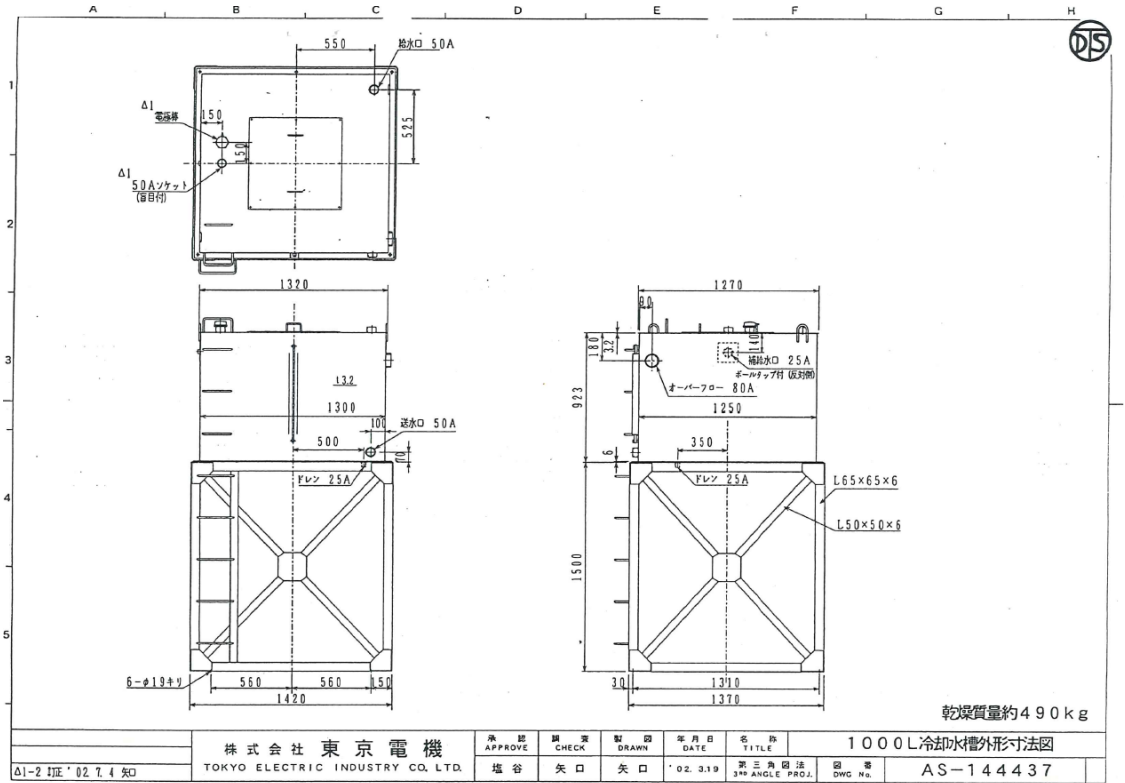
(2) エンジン用冷却水槽内部の姿図
