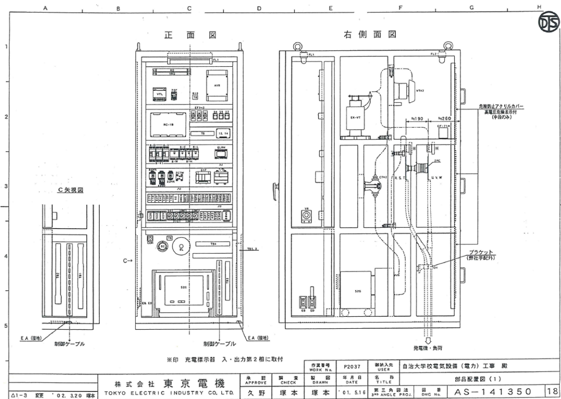
※発電機自動始動盤の姿図
