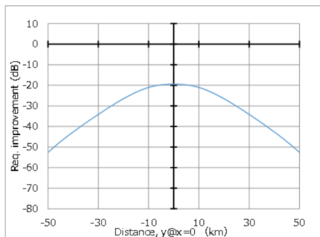
図 2. 4-9 与干渉：HAPS 局(Q 帯) (4)、被干渉：5G 移動局 (70 度指向)、同一周波数帯における共用検討結果 (STEP1)
