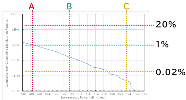
図 2. 5-19 与干渉：HAPS GW 局、被干渉：地球局、隣接周波数（100μW）における共用検討結果（STEP3）
