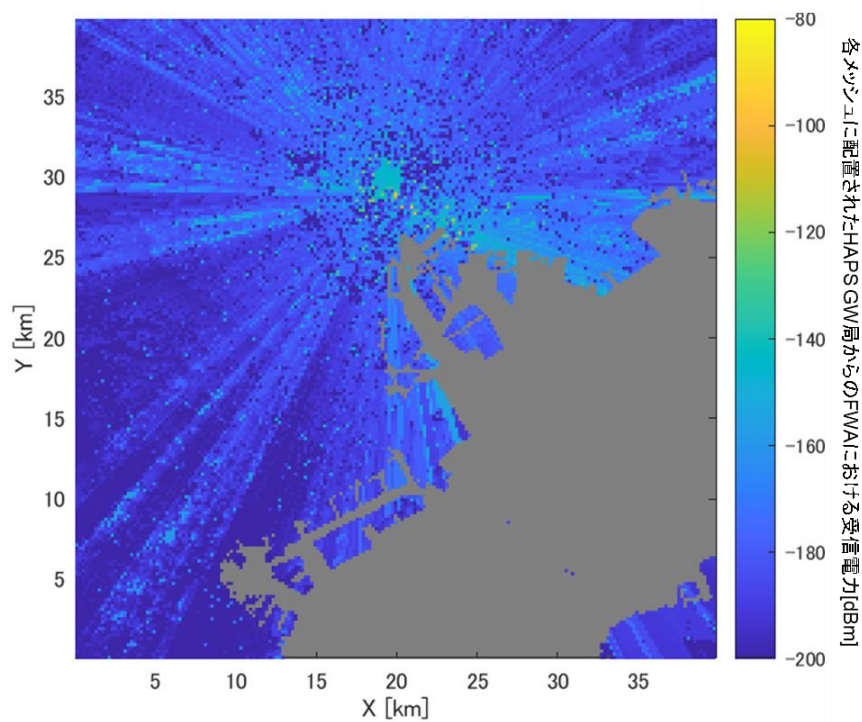
図 2. 1 1-1 7 HAPS GW 局から FWA への干渉電力分布 (STEP2)
