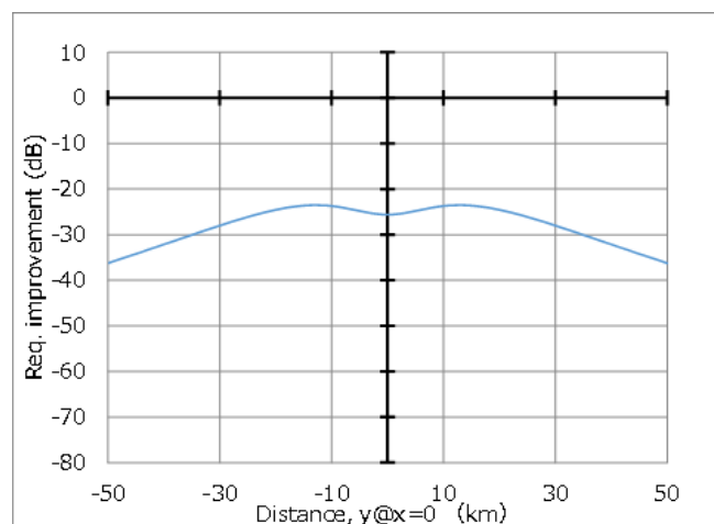
図 2. 4-10 与干渉：HAPS 局(Q 帯) (4)、被干渉：5G 移動局 (35 度指向)、同一周波数帯における共用検討結果 (STEP1)
