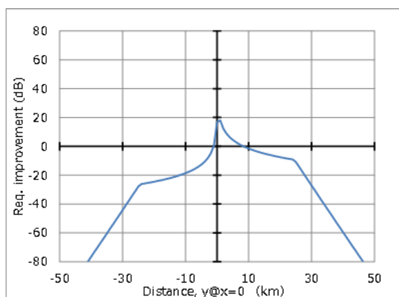
図 2. 6-4 与干渉: HAPS GW 局、被干渉: FWA 局、隣接周波数 (100 \mu W) における共用 検討結果 (STEP1)
