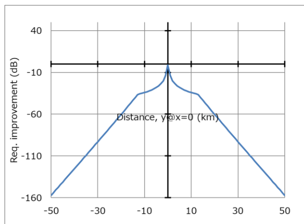
図 2. 4-3 9 被干渉：HAPS GW 局、与干渉：5G 移動局（メインビーム：35°）、隣接周波数（50μW）における共用検討結果（STEP1）
