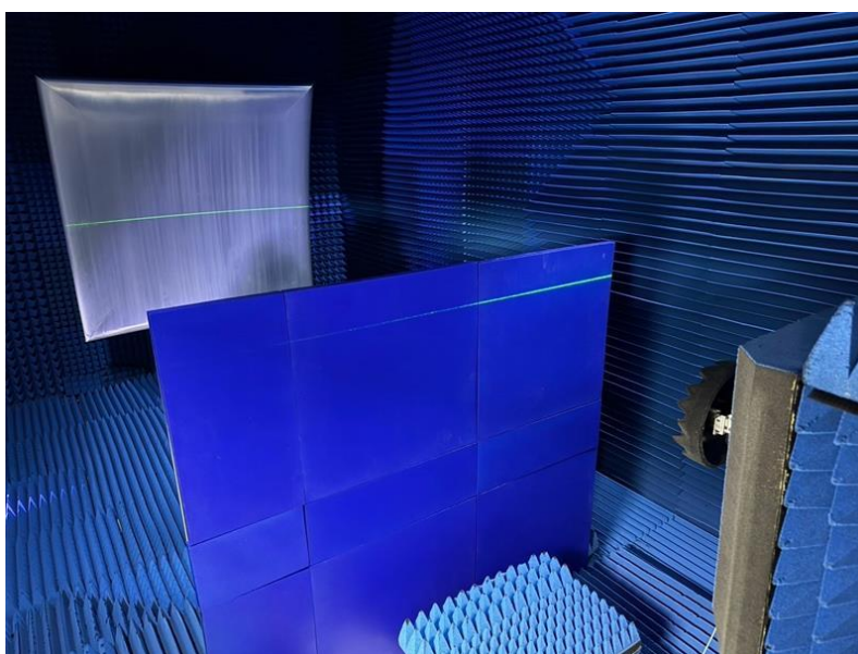
図 参 1. 2 - 1 Q 帯シールド減衰量測定試験の様子
