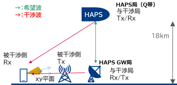
図 2. 4-8 STEP1 評価構成 (HAPS 局 (Q 帯)/HAPS GW 局が与干渉、5G 移動局が被干渉)
