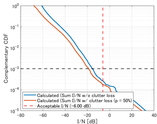
図 3. 7-4 与干渉：HAPS 局（S 帯）、被干渉：宇宙研究下り（2200～2290MHz）【Rx Gain = 56.3dBi】、隣接周波数（STEP3）（1:1 評価）
