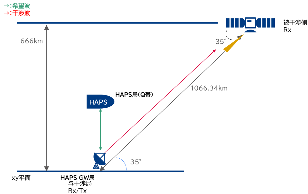
図 2. 7-1 STEP1 評価構成 (HAPS GW 局が与干渉、衛星受動センサが被干渉)
