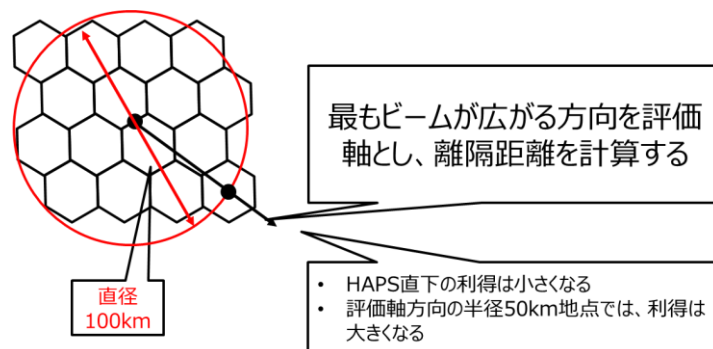
図 3. 2-1 HAPS 直下を中心に 16 ビームを六角格子状に配置するビーム配置
