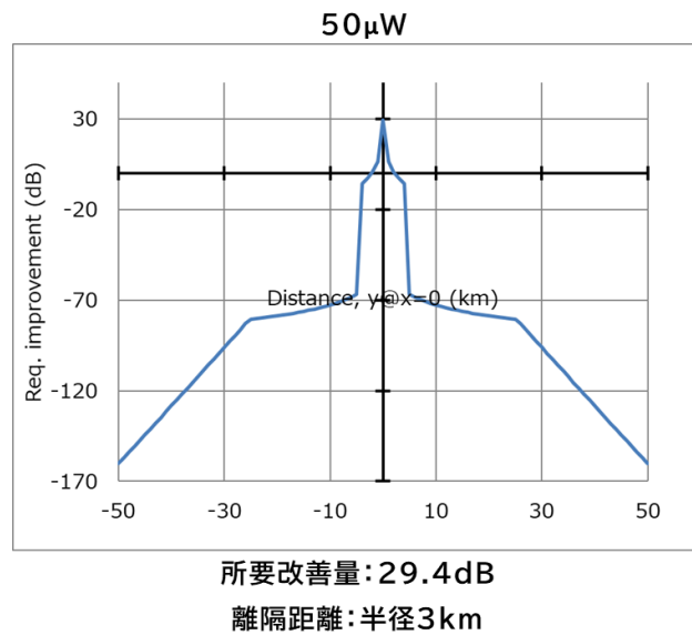
図 2. 6-38 被干渉: HAPS GW 局、与干渉: FWA、隣接周波数 (50μW) における共用検討結果 (STEP2)
