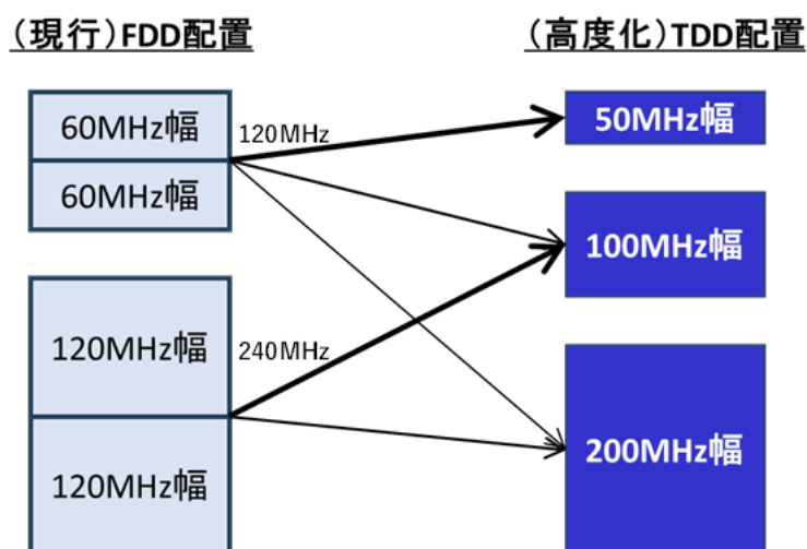
図 2-8 26GHz 帯から 22GHz 帯への移行イメージ
