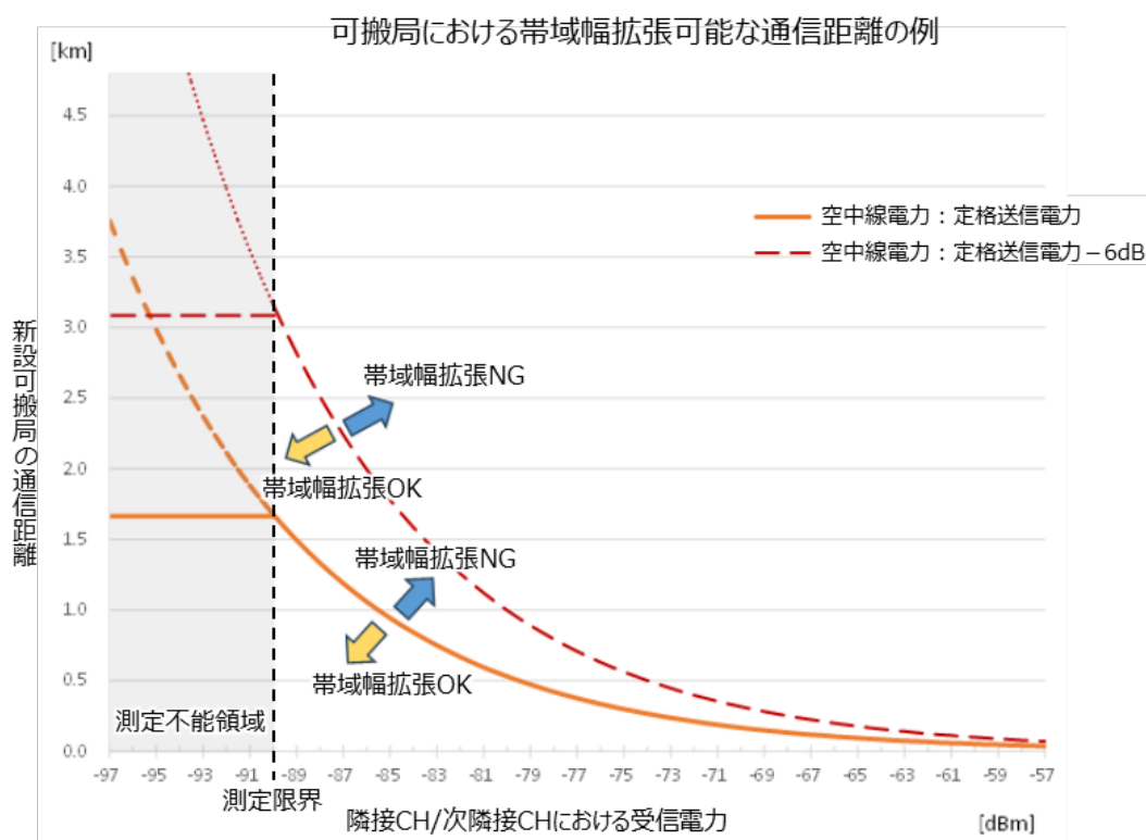
図 2-14 帯域幅拡張による干渉回避可能な許容通信容量装置 A の帯域幅拡張が装置 B へ干渉する場合の例
