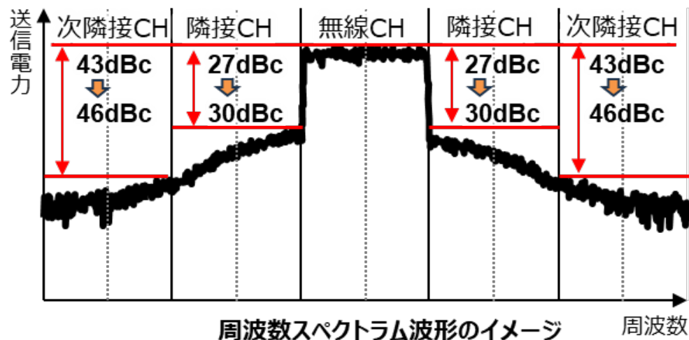
図 2-10 隣接チャネル漏えい電力の低減
