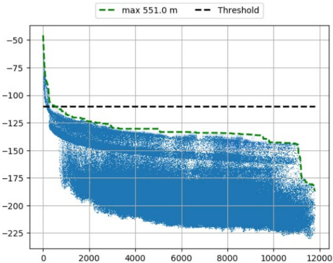
ゲートウェイ 1 (山地)、屋外 基地局最大パターン受信利得
