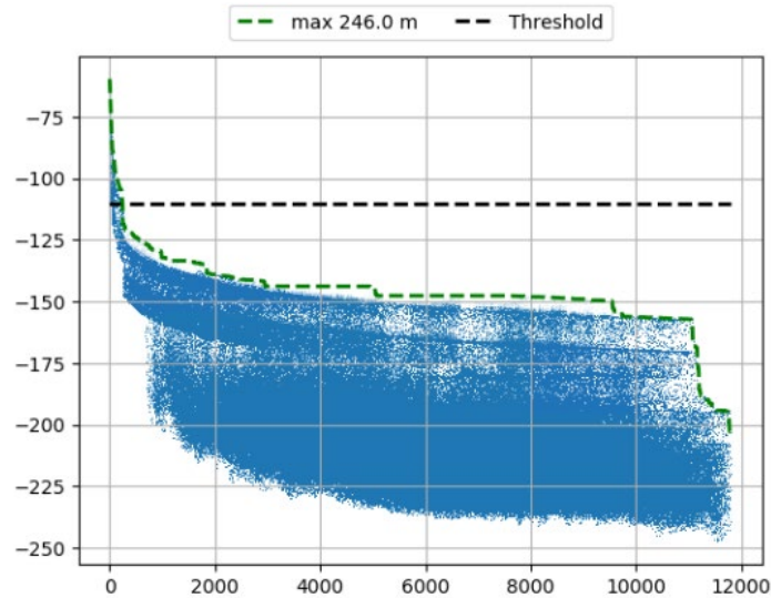
ゲートウェイ 1 (山地)、屋外 基地局平均パターン受信利得
