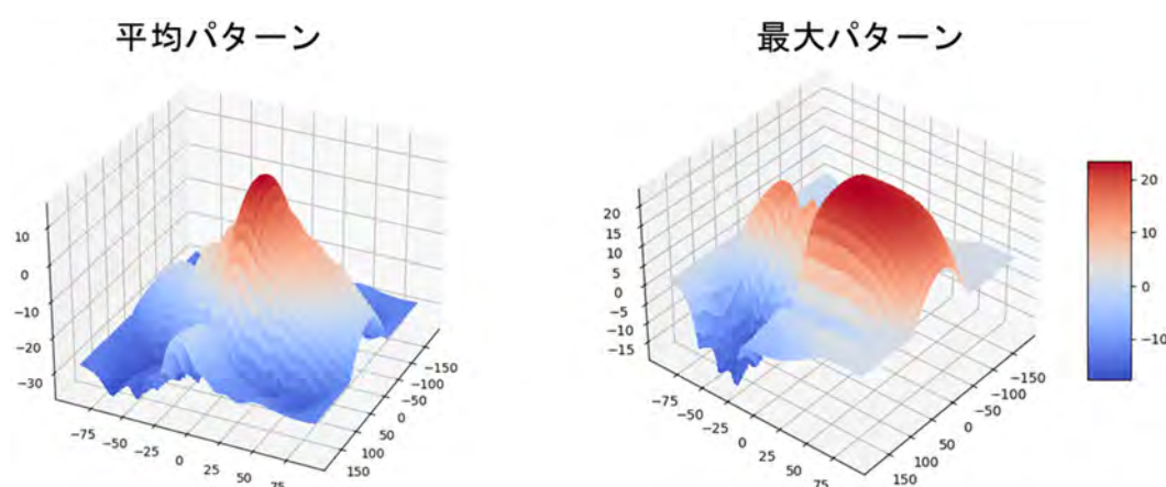
図 4. 2. 2-2 移動通信システム（ローカル 5 G）の基地局の空中線指向特性
