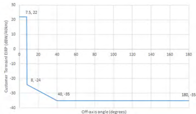
図 6. 2. 3-1 EIRP 密度（軸外）
