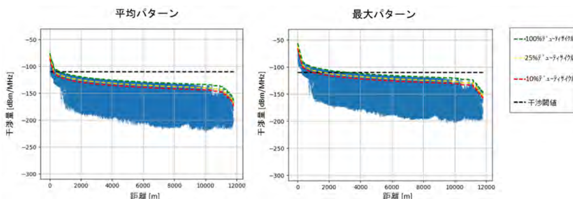
図 4. 2. 2-4 干渉検討結果（屋外設置、アンテナ高 10m、 郊外近郊 クラッタ考慮）
