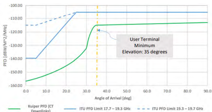
図 4. 1. 2-1 Ka 帯非静止衛星通信システム (600km) (衛星局) (ユーザー地球局対向) の PFD について
