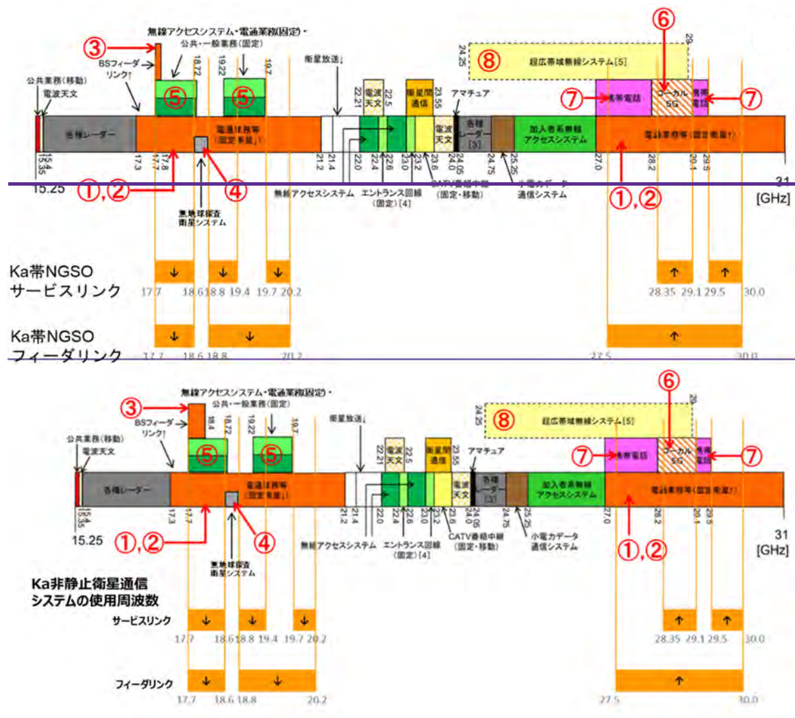
図 2. 1. 1-1 Ka 帯の周波数の利用状況
