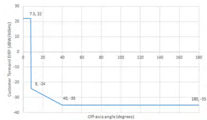
図 2. 3-1 EIRP 密度 (軸外)
