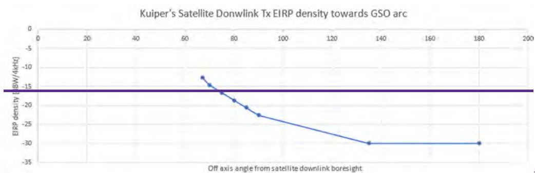
図2.3.3.2-3 Ka 帯非静止衛星通信システム（衛星局）のEIRP 密度（参考）
