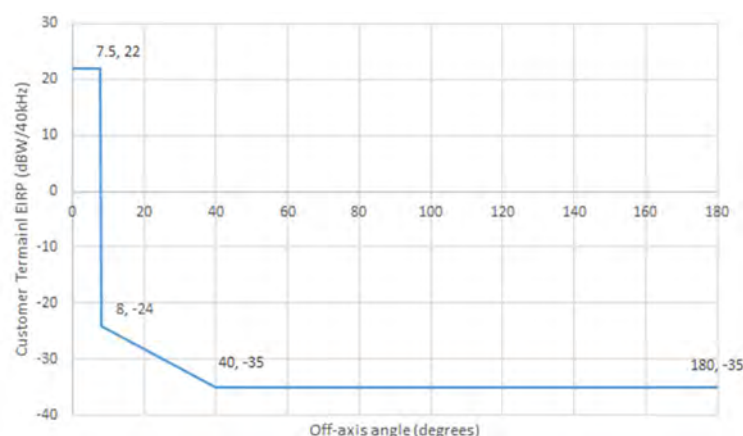
図 2. 3. 1－1 Ka 帯非静止衛星通信システム（ユーザー地球局）の EIRP 密度（軸外）
