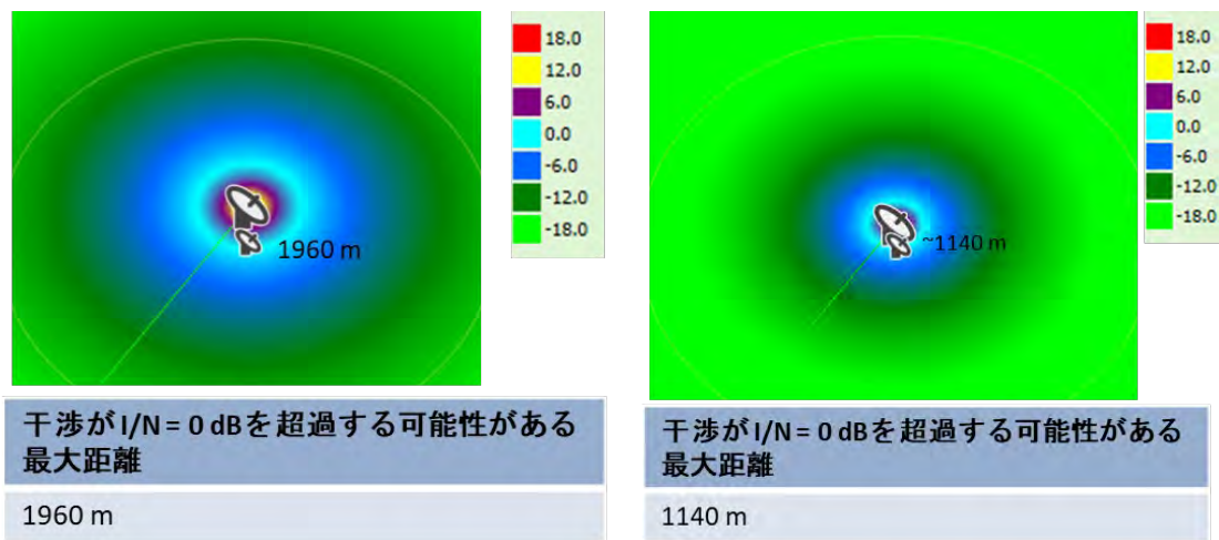
(a) 被干渉局がユーザー局の場合
