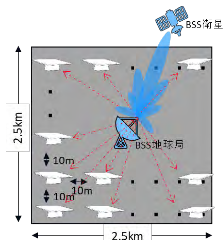
図 3. 3. 3-1 評価のモデル
