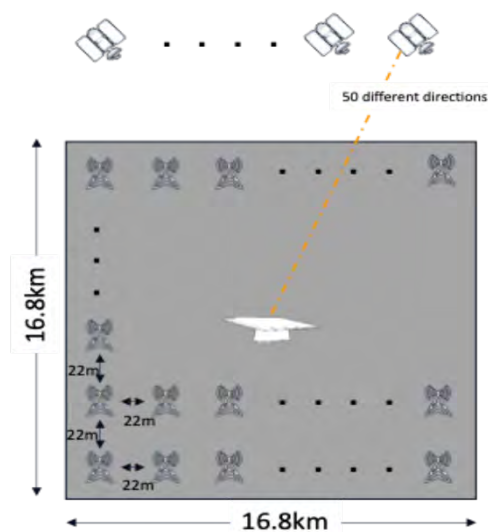
図 4. 2. 2-1 共用検討のモデル
