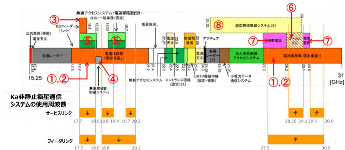
図 2. 1. 1-1 Ka 帯の周波数の利用状況
