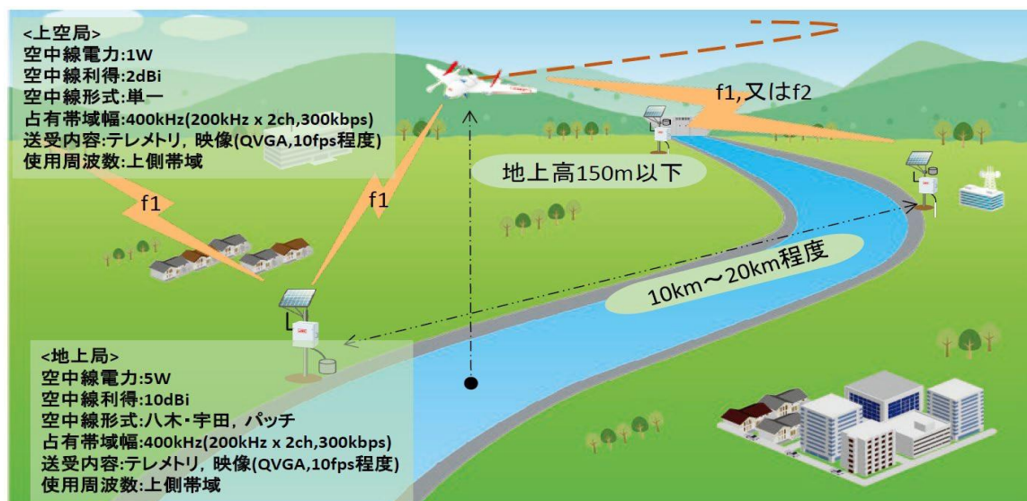
図 10 災害対応 IoT 無線利用 (UAV 等機械制御 (ドローン利用)) の利用イメージ例
