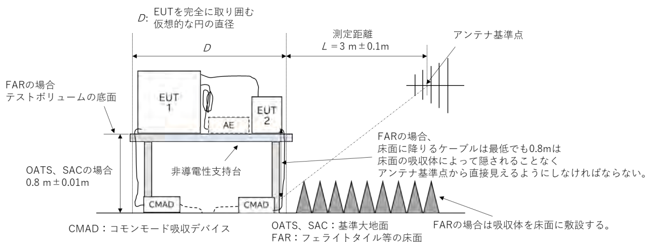
図 3b 側面図
