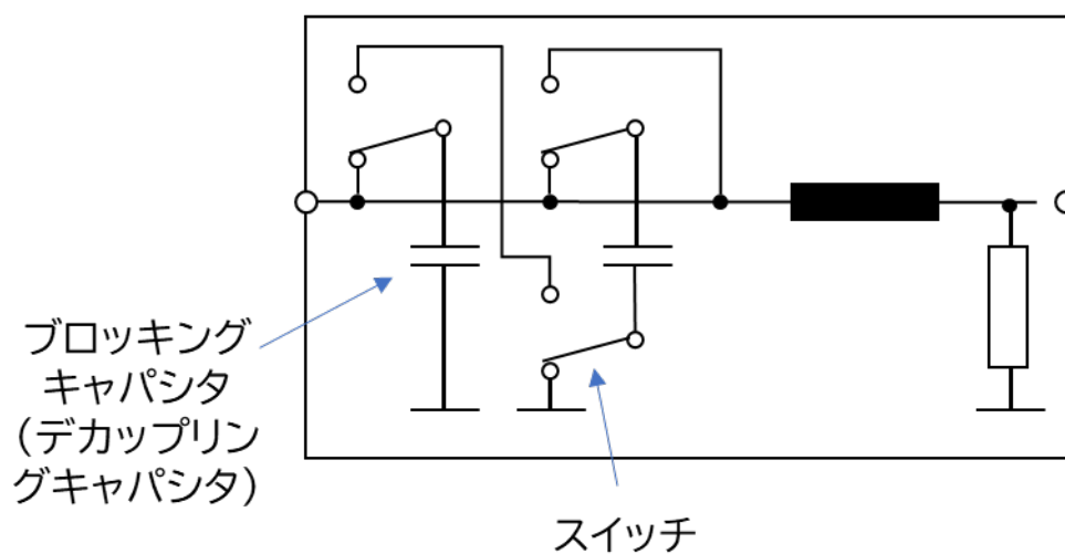
図 E.7 LC デカップリング回路のブロッキングキャパシタの静電容量を増減可能な DC-AN 回路例
