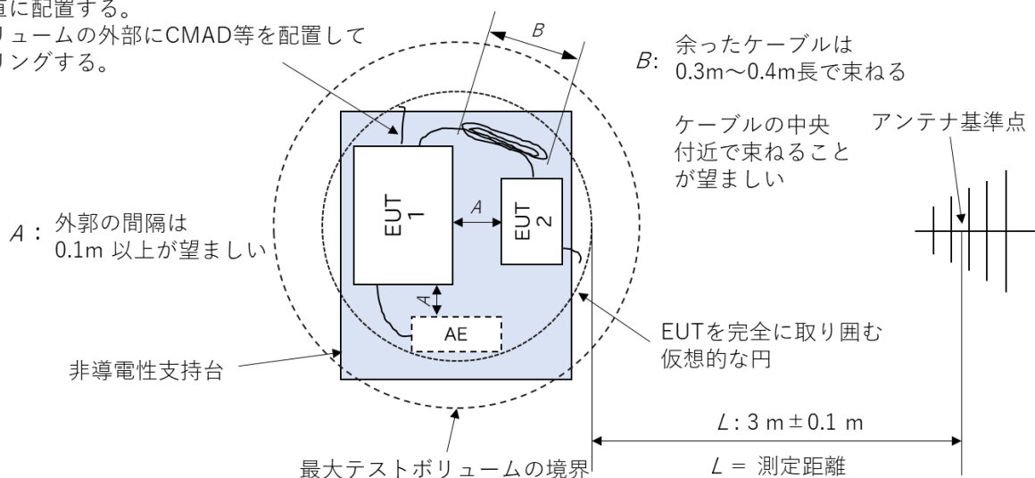
図 3a 上面図
