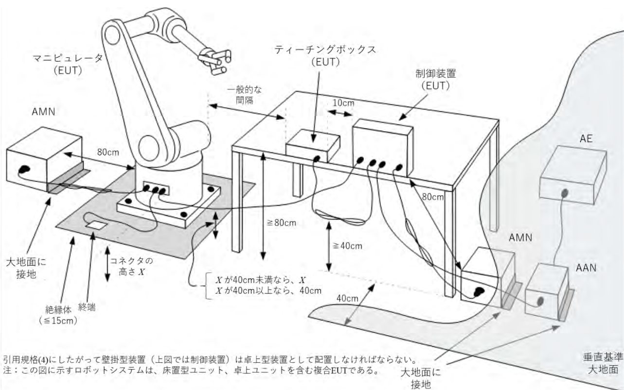
図 8 複合ロボットシステムの伝導妨害波測定における一般的配置例
