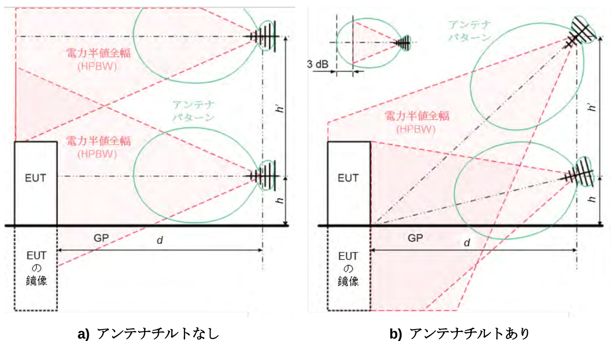
図 F.4 - アンテナ指向性の影響
