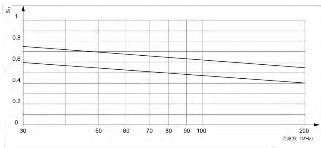
図 28 - 8.1 節から 8.3 節に基づいて測定された S_{11} の絶対値の許容範囲
