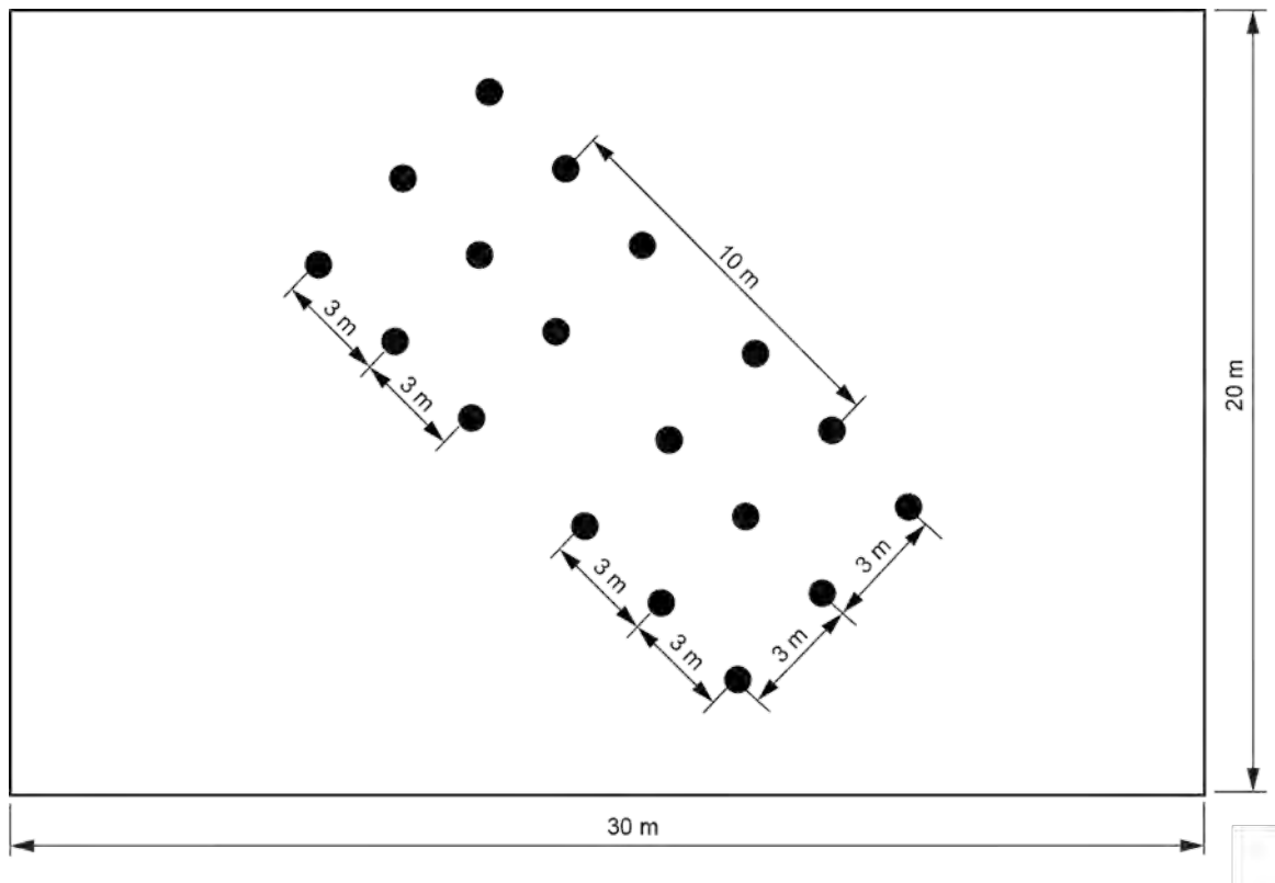
図 9 - 10 m のテスト距離のペアテスト箇所の選択の例
