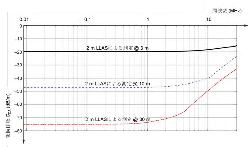
図 C.11 - 三つの測定距離 d に関する変換係数 C_{dA} \text{dB}(\mu\text{A}/\text{m}) への変換
