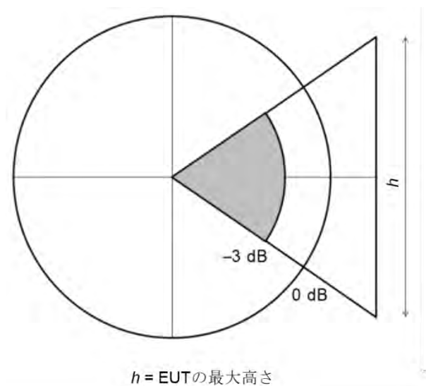
図 4 - アンテナの半値幅を用いた適用可能な EUT の最大高さの決定
