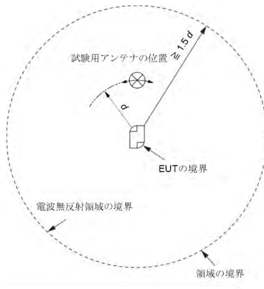
図 6 - 据え置き EUT における電波無反射領域
