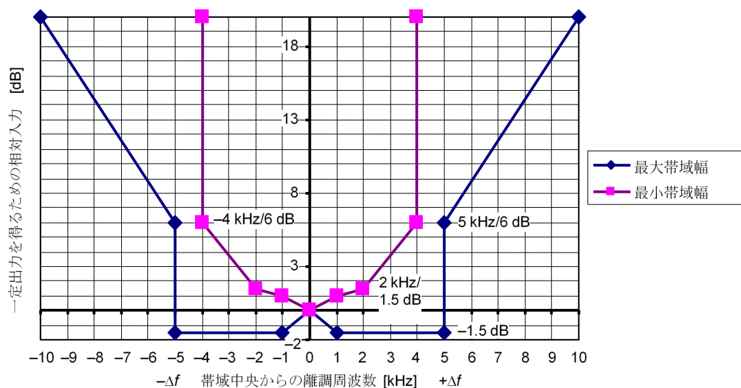
図 2 - 総合選択度の許容範囲ー通過帯域 (バンド B)
