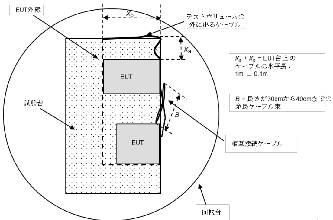
図 16 - 卓上型装置の試験配置
