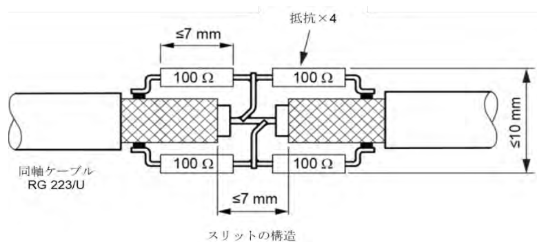
図 C.2 - 電流プローブと対称に配置された二つの向かい合うスリットを持つ LLA
