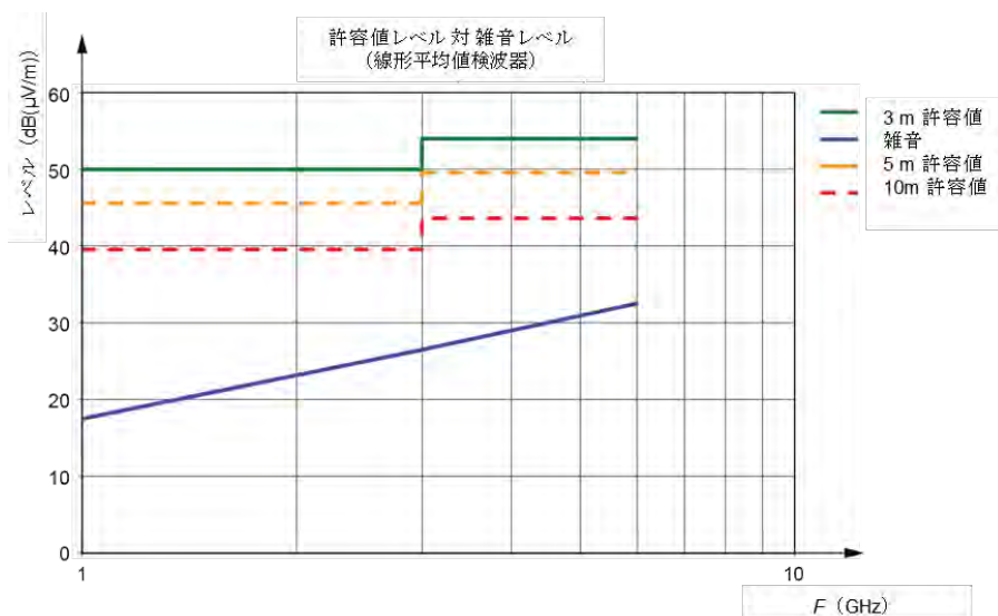
図 F.7 - 周波数範囲 1 GHz から 6 GHz で 3 m、5 m、及び 10 m の距離の線形平均値検波器の妨害波許容値 E_{Lav} と比較したノイズレベル E_{Nlogav} (例: 10 \log F_{tot} = 4 \text{ dB} )
