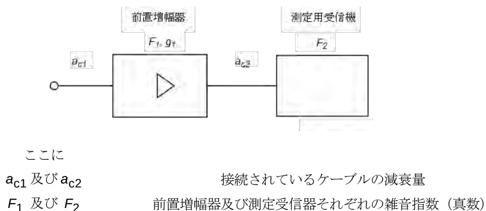
図 A.3 - システム雑音指数の説明図
