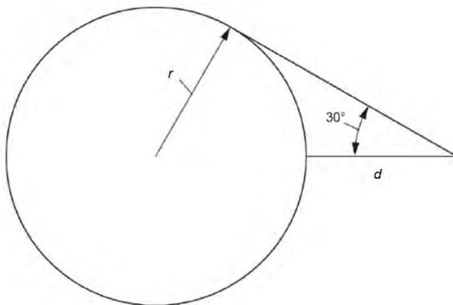
図 F.3 - 特定の距離 d とアンテナビーム幅 60^\circ でのテストボリュームの半径 r
