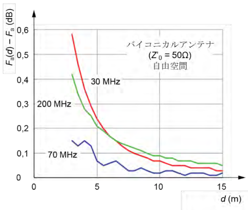
図 F.2 - バイコニカルアンテナの自由空間 AF からの近傍界 AF の偏差 (参考文献 [2] の図 C.5.b)
