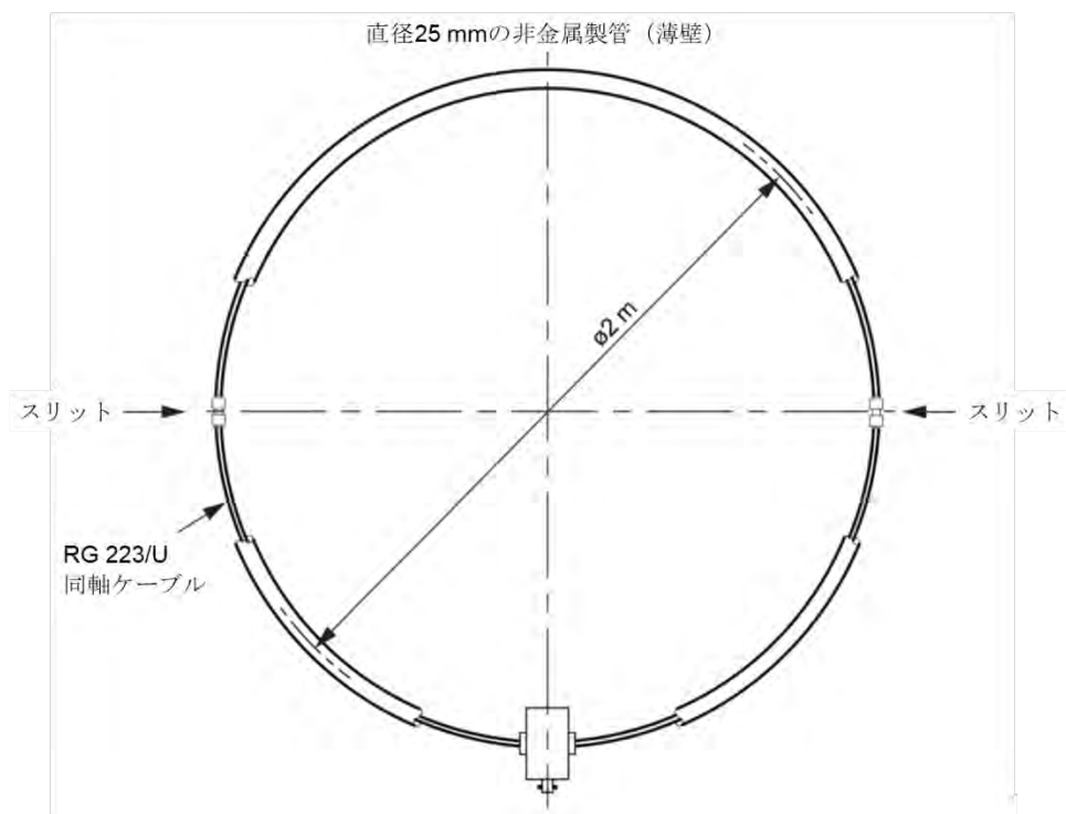
図 C.2 - 電流プローブと対称に配置された二つの向かい合うスリットを持つ LLA
