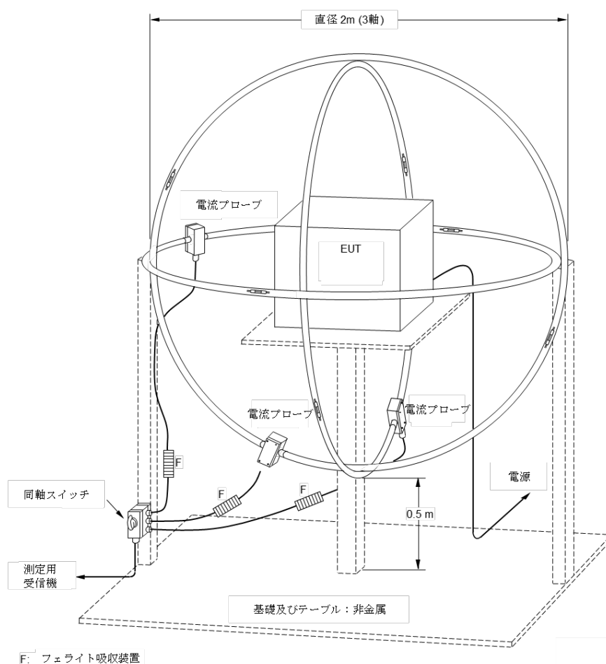
図 7 - LLAS を用いた磁界誘導電流測定概念
