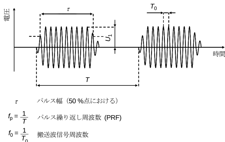
図 E.4 - 測定用受信器に輸入されるパルス変調 RF 信号
