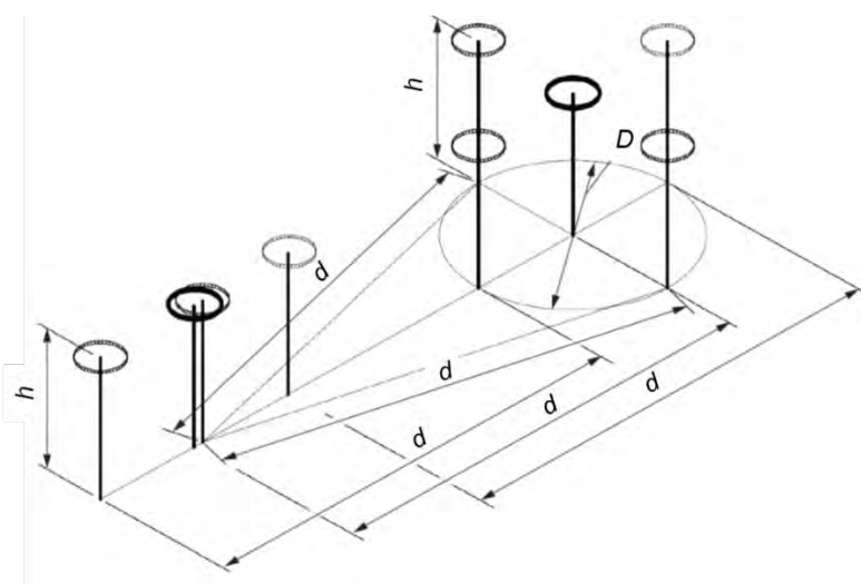
c) ループアンテナを用いた H_z の妥当性確認
