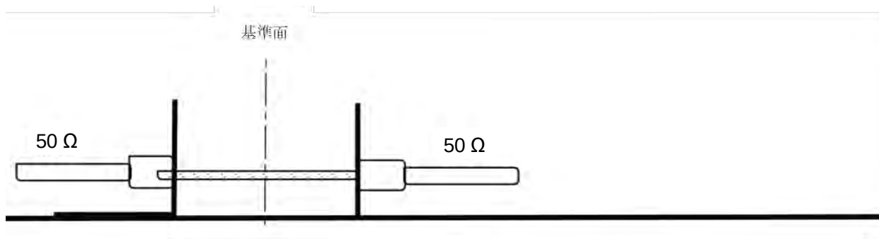
図 27c - 「通過」の校正測定系の構成
