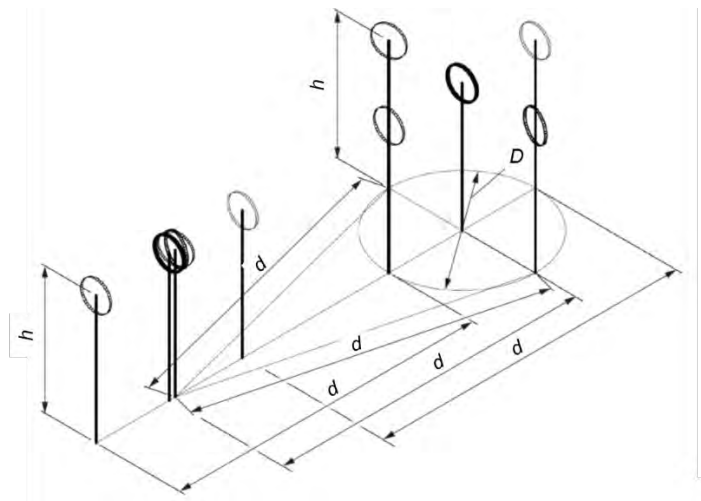
a) ループアンテナを用いた H_x の妥当性確認
