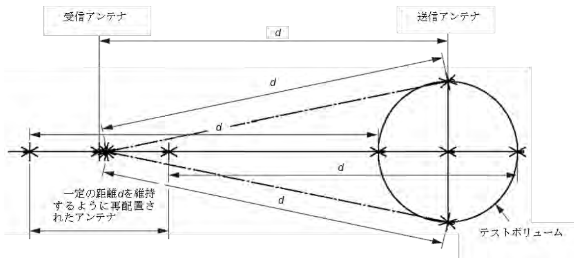
図 11 - 全天候型 OATS 及び SAC における典型的なアンテナ配置 垂直偏波妥当性確認測定
