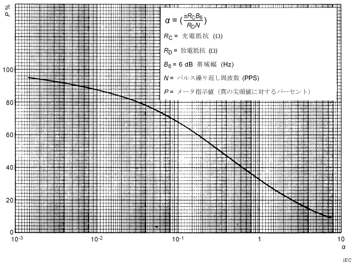
図 E.2 - 繰り返しパルスに対する検波効率 P
