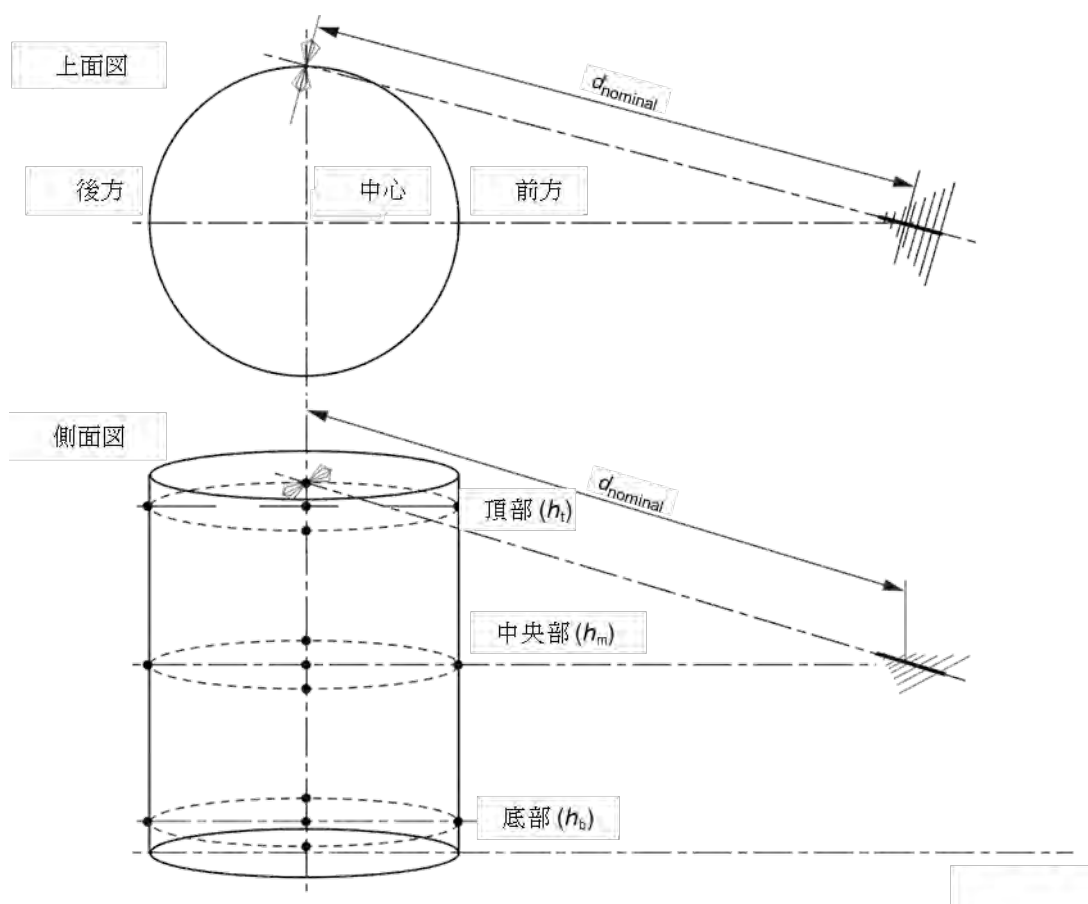
図 16 - FAR 試験場妥当性確認のための一つの測定位置及びアンテナ傾斜の例
