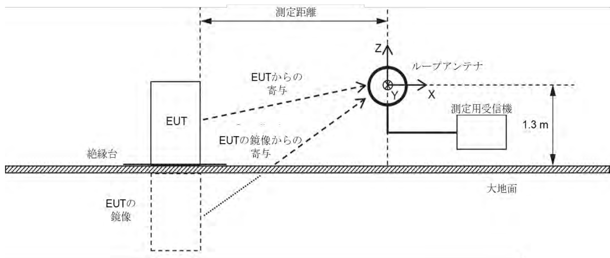
図 26 - OATS 又は SAC における床置型 EUT の磁界強度測定セットアップの概念
