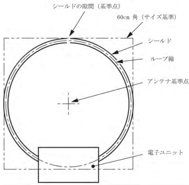
図 34 - サイズ基準に準拠したループアンテナの例
