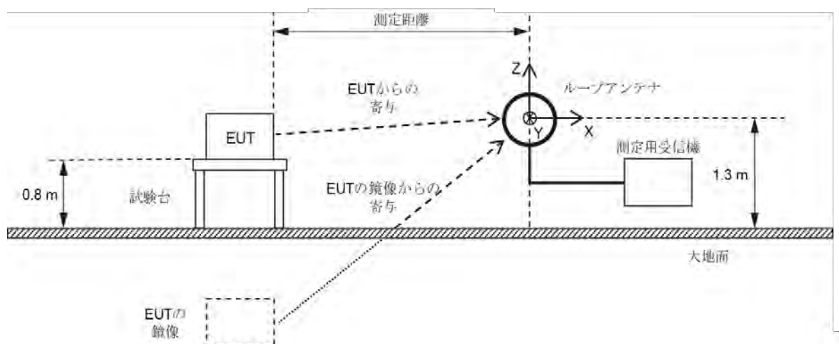
図 25 - OATS 又は SAC における卓上型 EUT の磁界強度測定セットアップの概念
