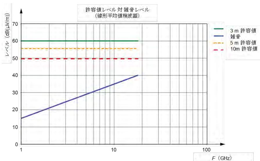
図 F.8 - 周波数範囲 1 GHz から 18 GHz で 3 m、5 m、及び 10 m の距離の対数平均値検波器の妨害波許容値 E_{Lav} と比較したノイズレベル E_{Nlogav} (例: 10 \log F_{tot} = 4 \text{ dB} )
