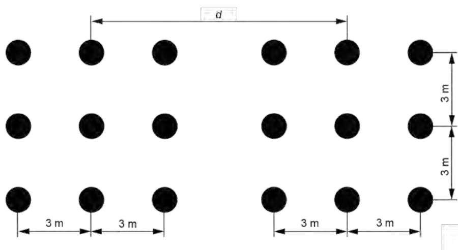
図 8 - 全テスト距離のペアテスト箇所の場合
