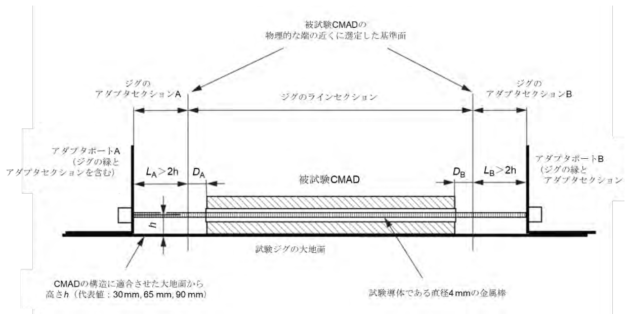
図 26 - 試験ジグ内部の基準面の定義
