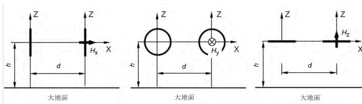
図 35 - 一般的なアンテナの三つの向き H_x, H_y 及び H_z ( d は測定距離、 h はアンテナの基準点の高さ)
