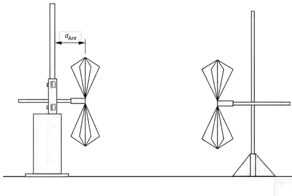
図 10 - A_{APR} に関するアンテナポジションの影響の調査の図
