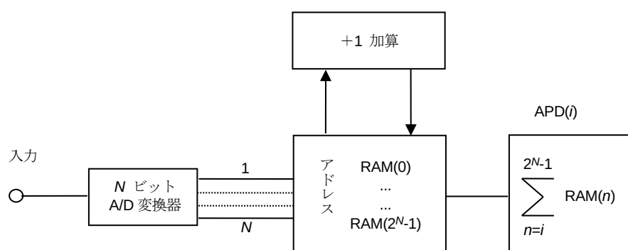
図 G.2 - A/D 変換器を使用する APD 測定回路のブロック図
