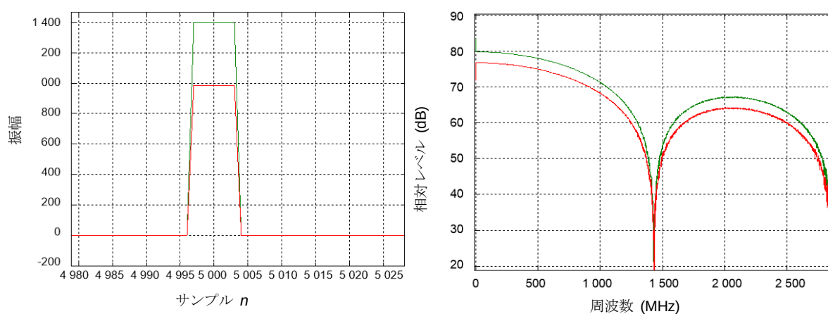
図 J.3 - 正弦波信号に対する図 J.2 に示す伝達関数を持つ増幅器の応答
