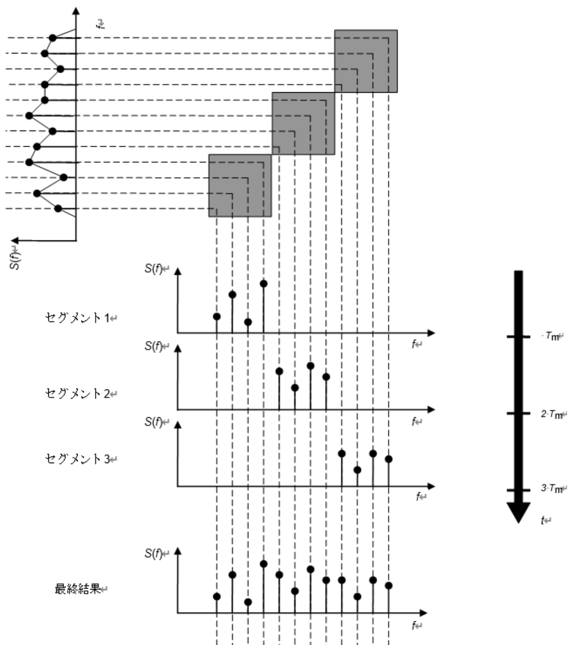
図 5 - セグメントごとの FFT 走査
