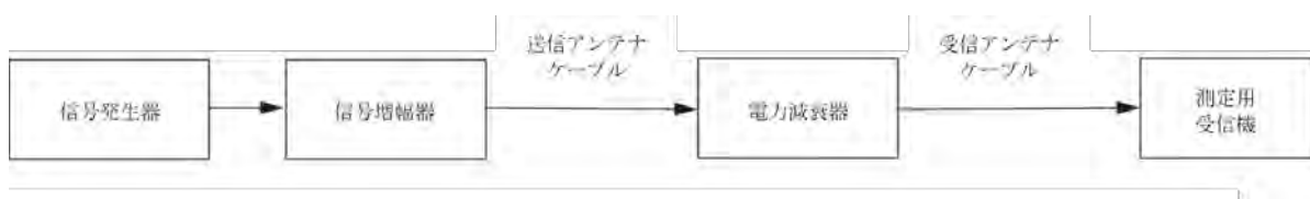
図 38 - 電力増幅器と減衰器を用いた V_{\text{DIRECT}} の測定構成
