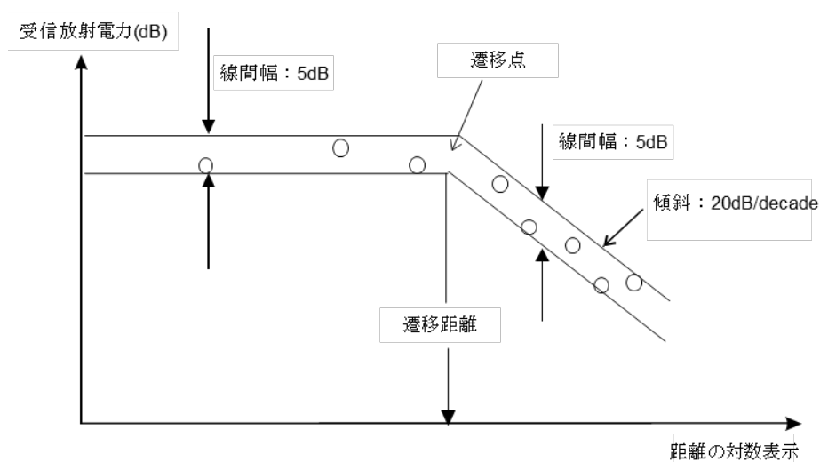
図 22 - 遷移距離の決定
