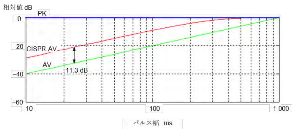
図 C.4 - 尖頭値“PK”と平均値に対する重み付け関数の計算例 (繰り返し周波数 1 Hz、指示計の機械的時定数 100 ms)
