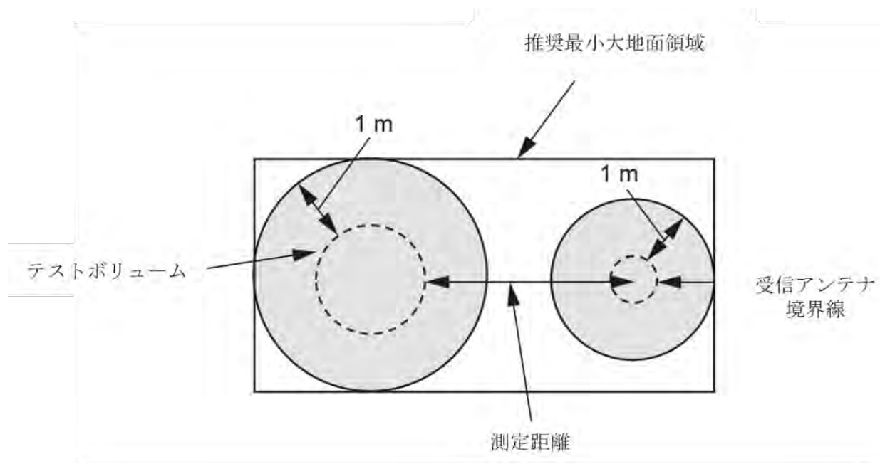
図 K.1 - 大地面の推奨最小寸法（上面図）
