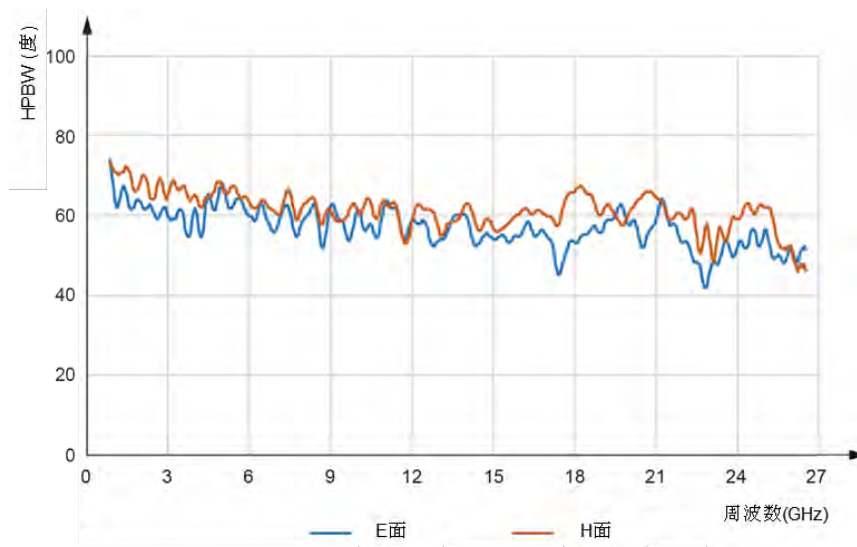
図 F.5 - V 型 LPDA アンテナの HPBW (E 面 / H 面)
