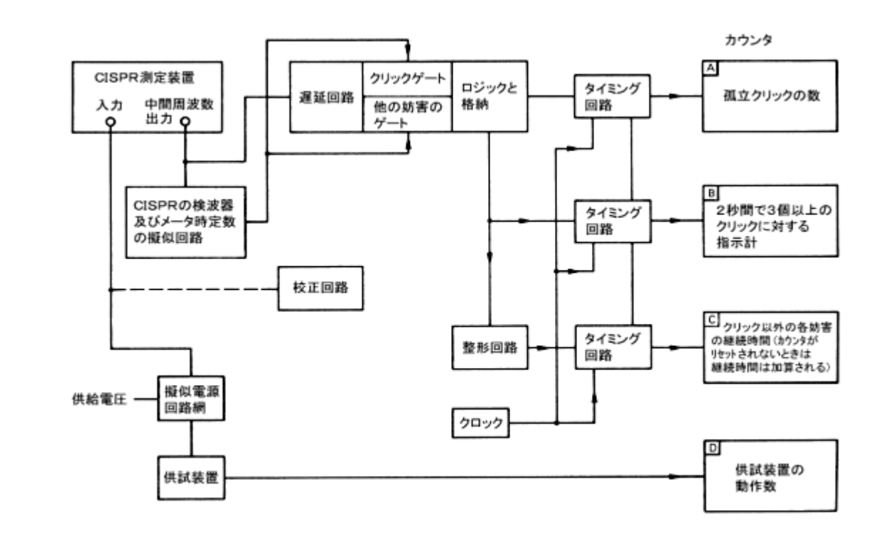
図 12 - 不連続性妨害波アナライザの例
