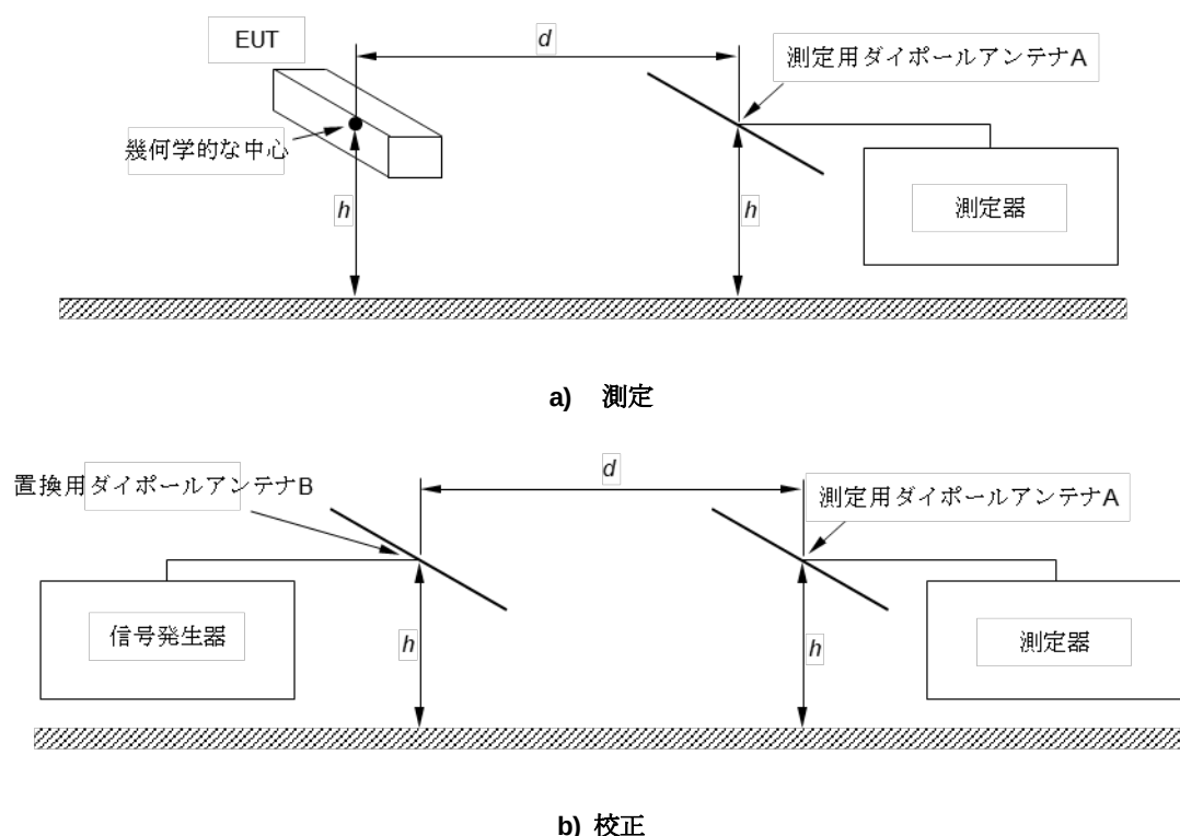
図 23 - 置換法による測定配置構成 : a) 測定、b) 校正
