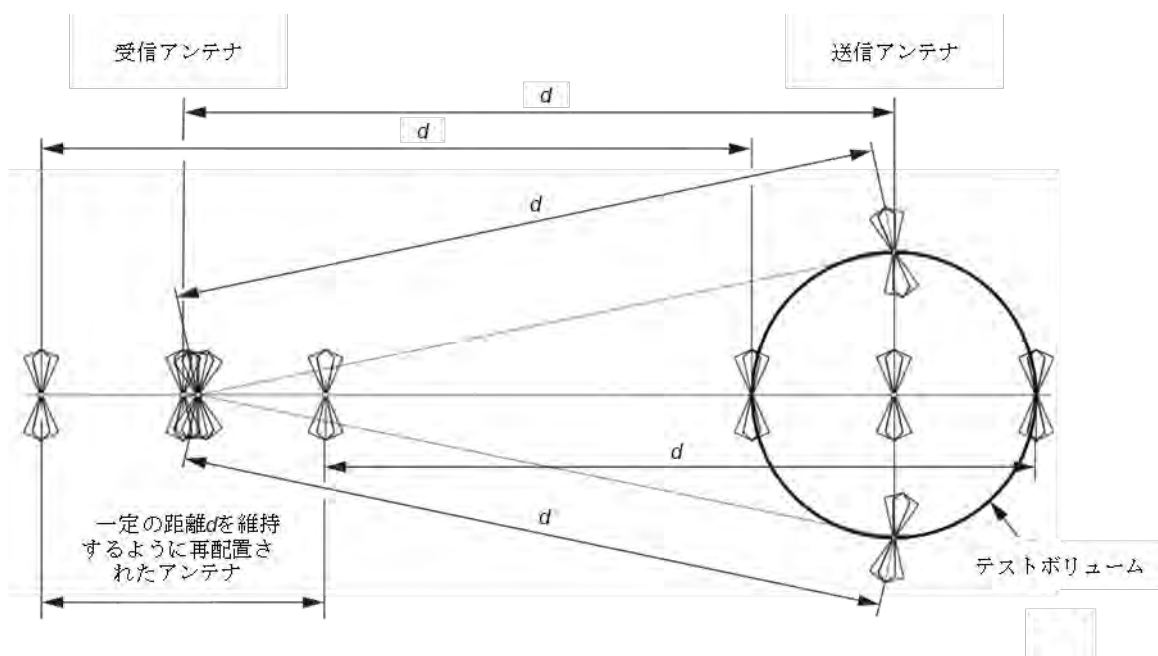
図 12 - 全天候型 OATS 及び SAC における典型的なアンテナ配置 水平偏波妥当性確認測定
