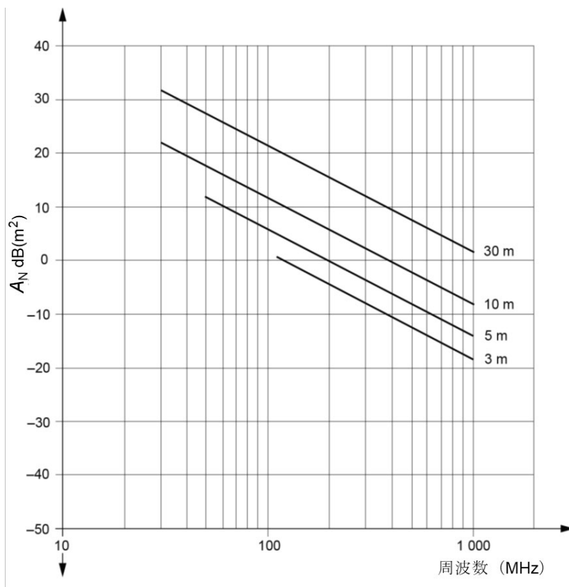
図 18 - 異なる測定距離に対する周波数の関数としての自由空間 NSA の理論値 (式 (16) 参照)
