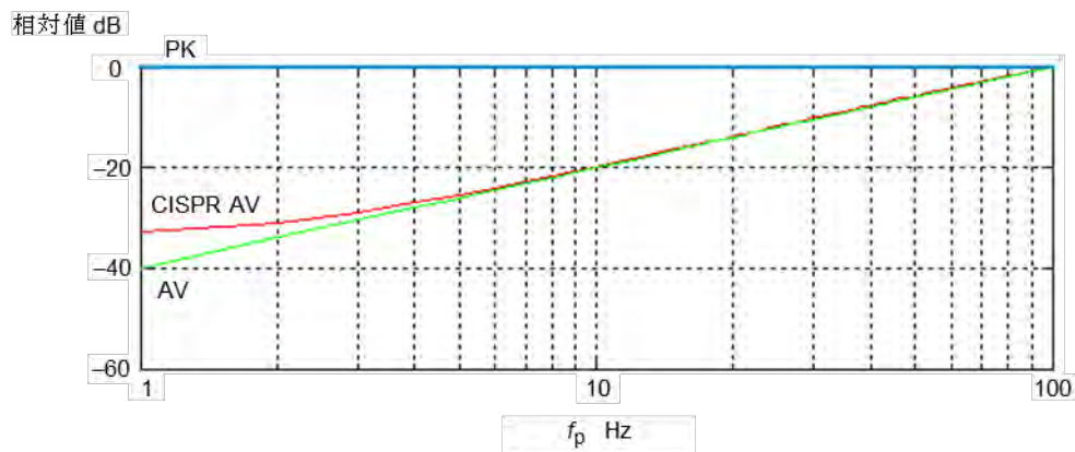
図 C.1 - 幅 10 ms のパルスに関する指示計の重み付け関数
