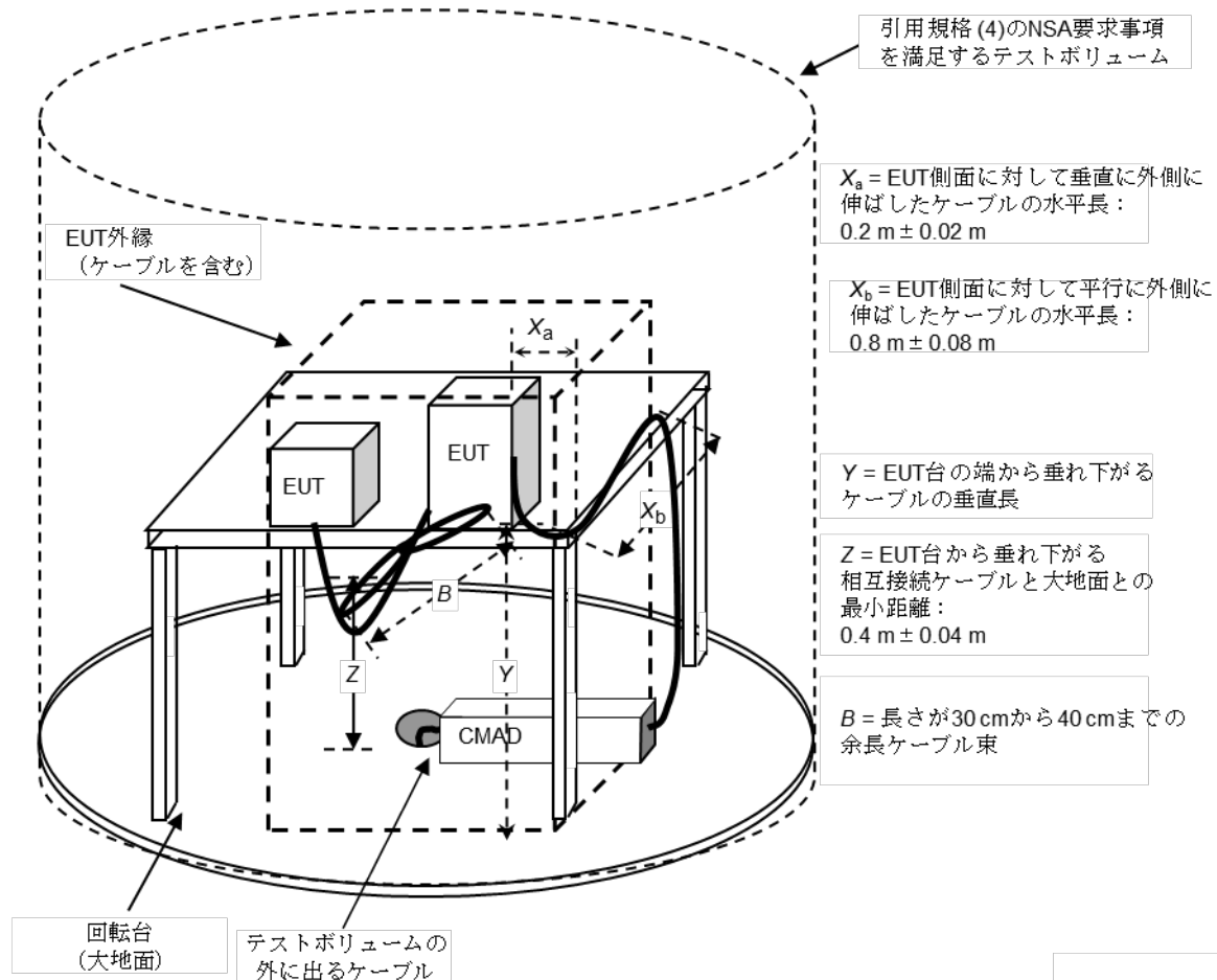
図 16 - 卓上型装置の試験配置
