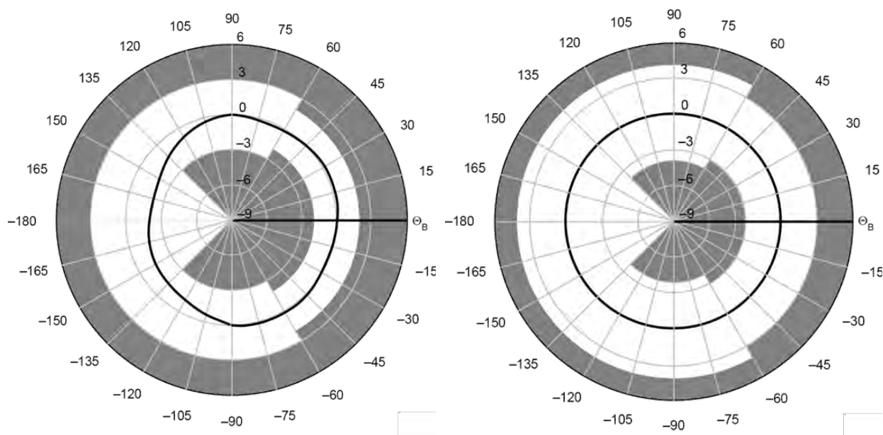
図 22a - 1 GHz から 6 GHz の放射パターンの例
