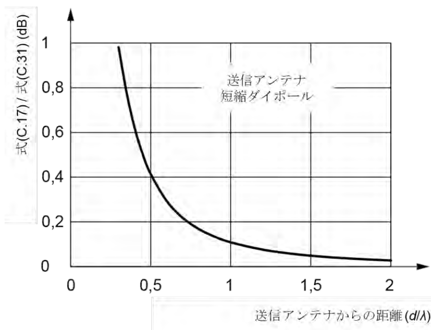
図 F.1 - 参考文献 [2] の式 (C.17)と参考文献 [2] の式 (C.31) による近傍界領域の比較
