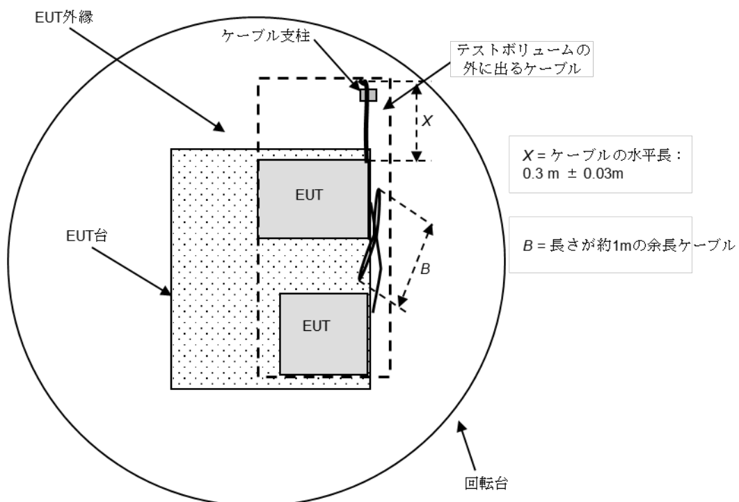
図 18 - 床置き型装置の試験配置
