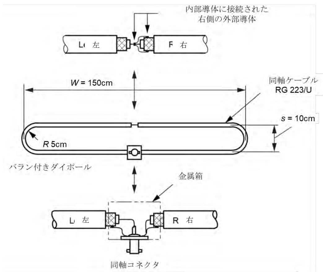
図 C.9 - バラン付きダイポールの構造
