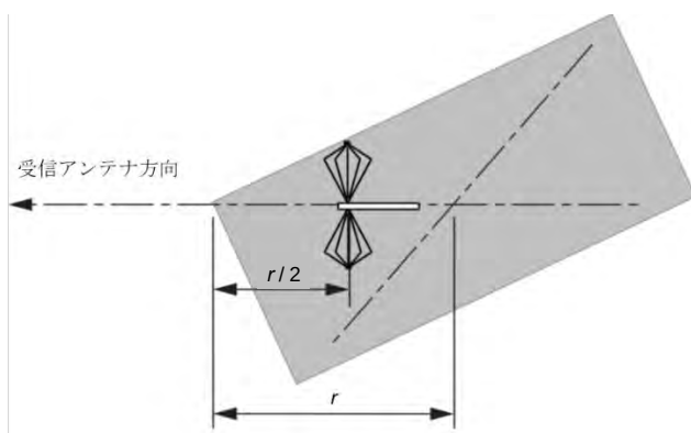
図 19 - 長方形試験台の角からのアンテナ配置 (平面図)
