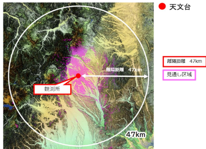
図参 4. 2. 5 自由学園那須農場電波観測所における空間伝送型ワイヤレス電力伝送システムの制限区域
