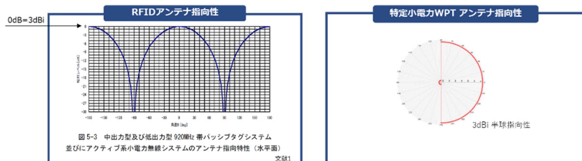
図参 4.1.1 RFID 特定小電力無線局との指向性差 ※11
