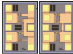
図 1.2.5 920MHz 帯 微弱電力対応整流器※3
