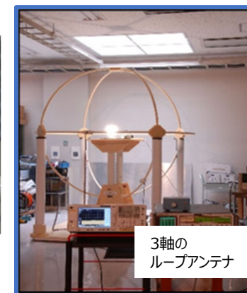
3軸の ループアンテナ システム (30MHz未満の妨害波 測定で使用)
