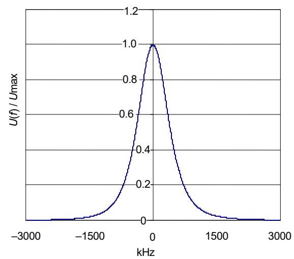
図 E.8 - 正規化された選択度特性 U(f) / U_{\max} の例 (1 MHz の場合)
