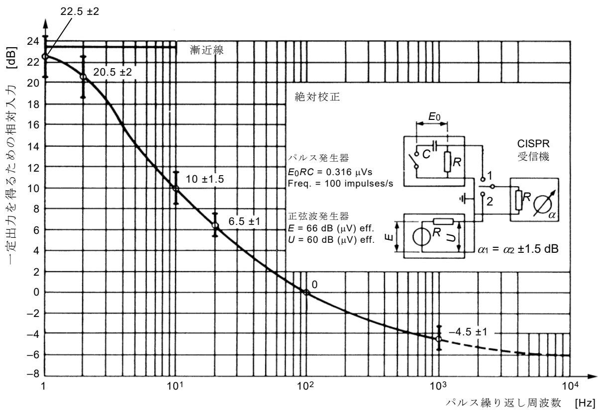
図 7 - パルス応答曲線 (バンド B)
