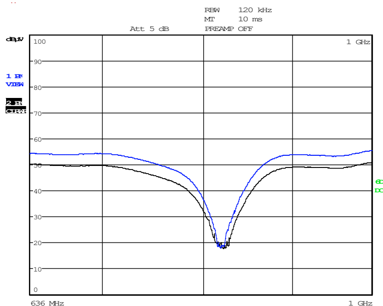
図 J.7 - 前置増幅器に対する 818 MHz 付近の帯域阻止フィルタ試験のスクリーンショット
