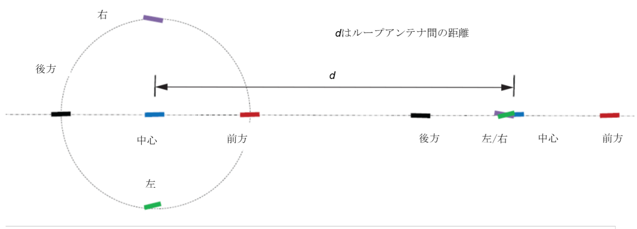
b) ループアンテナを用いた H_y の妥当性確認
