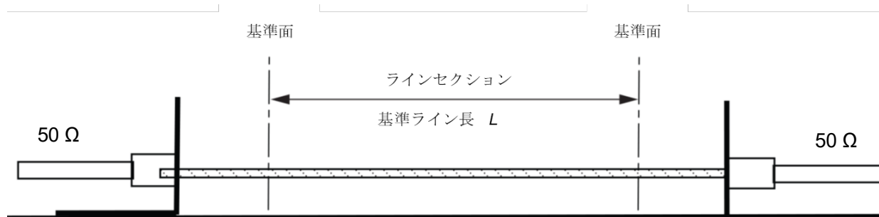
図 27c - 「通過」の校正測定系の構成
