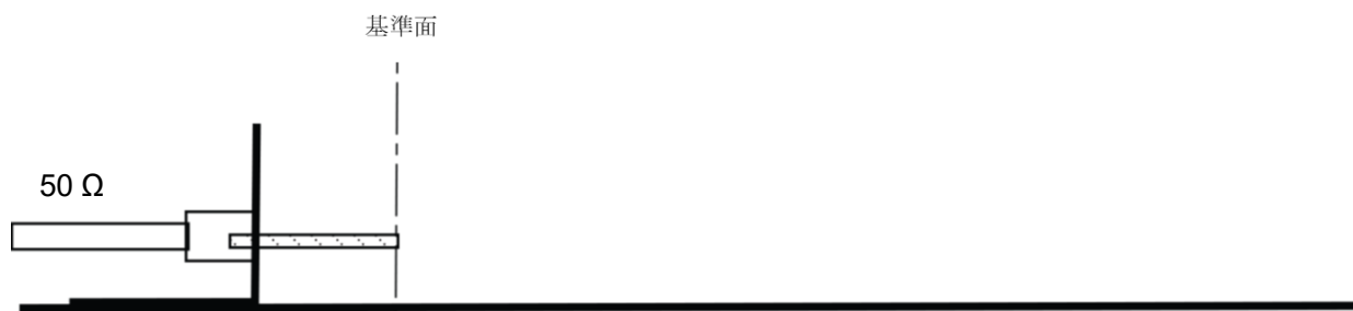
図 27a - 「反射」(ポート A) の校正測定系の構成
