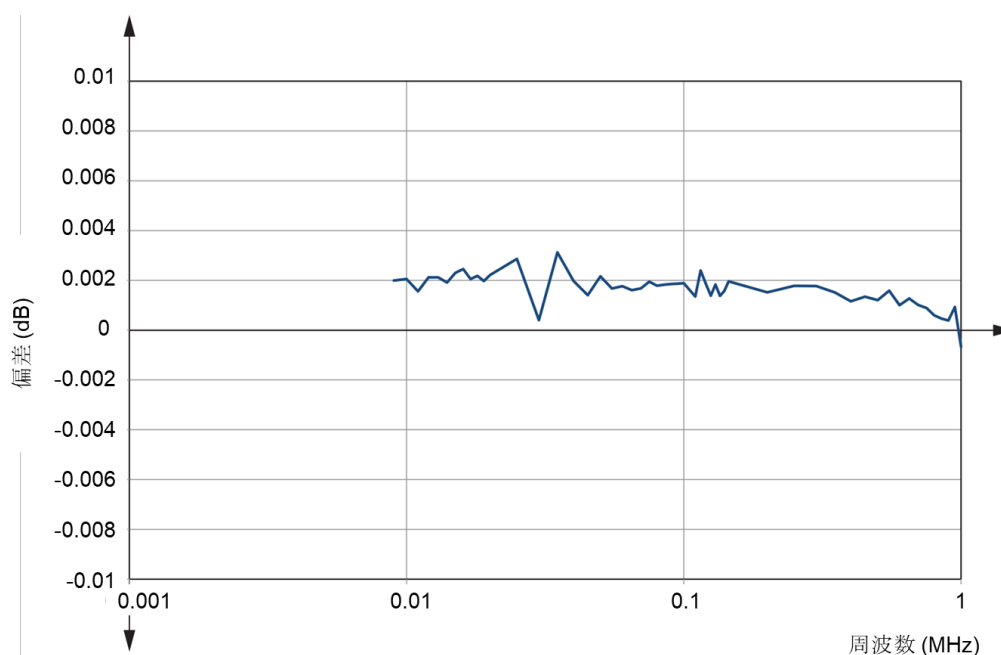
図 L.1 – 解析式とコンピュータシミュレーションによる NSIL 値の比較
