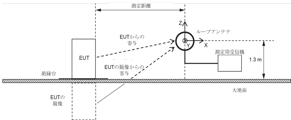
図 26 - OATS 又は SAC における床置型 EUT の磁界強度測定セットアップの概念
