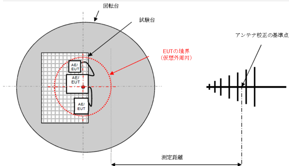
図 8 - 測定距離
