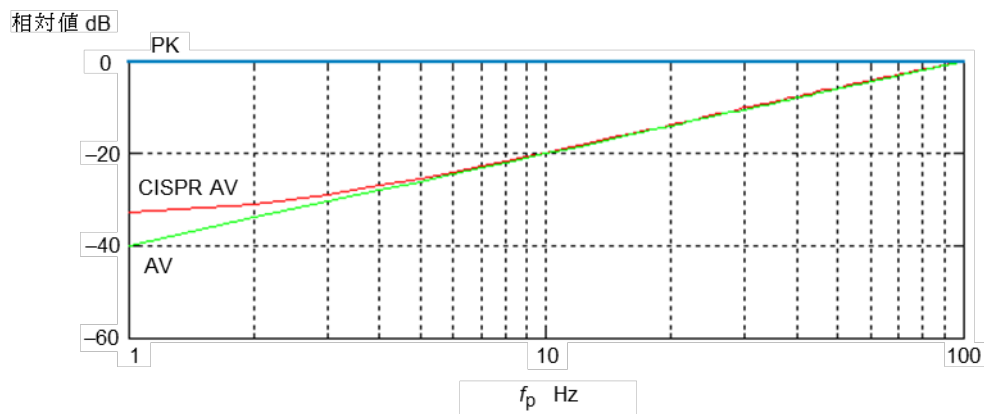
図 C.1 - 幅 10 \text{ ms} のパルスに関する指示計の重み付け関数
