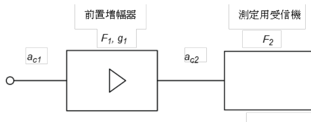
図 F.6 - 前置増幅器付き測定用受信機
