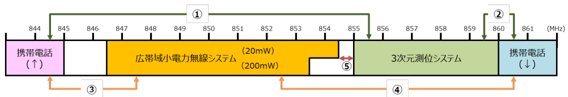
図 3.1-2 新システムの周波数配置のイメージ及び 共用検討の組合せ (デジタル MCA サービス終了後を想定)
