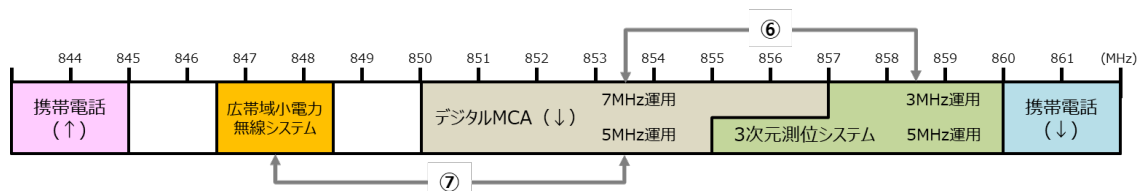
図 3.1-3 新システムの周波数配置のイメージ及び 共用検討の組合せ (デジタル MCA サービス期間中を想定)
