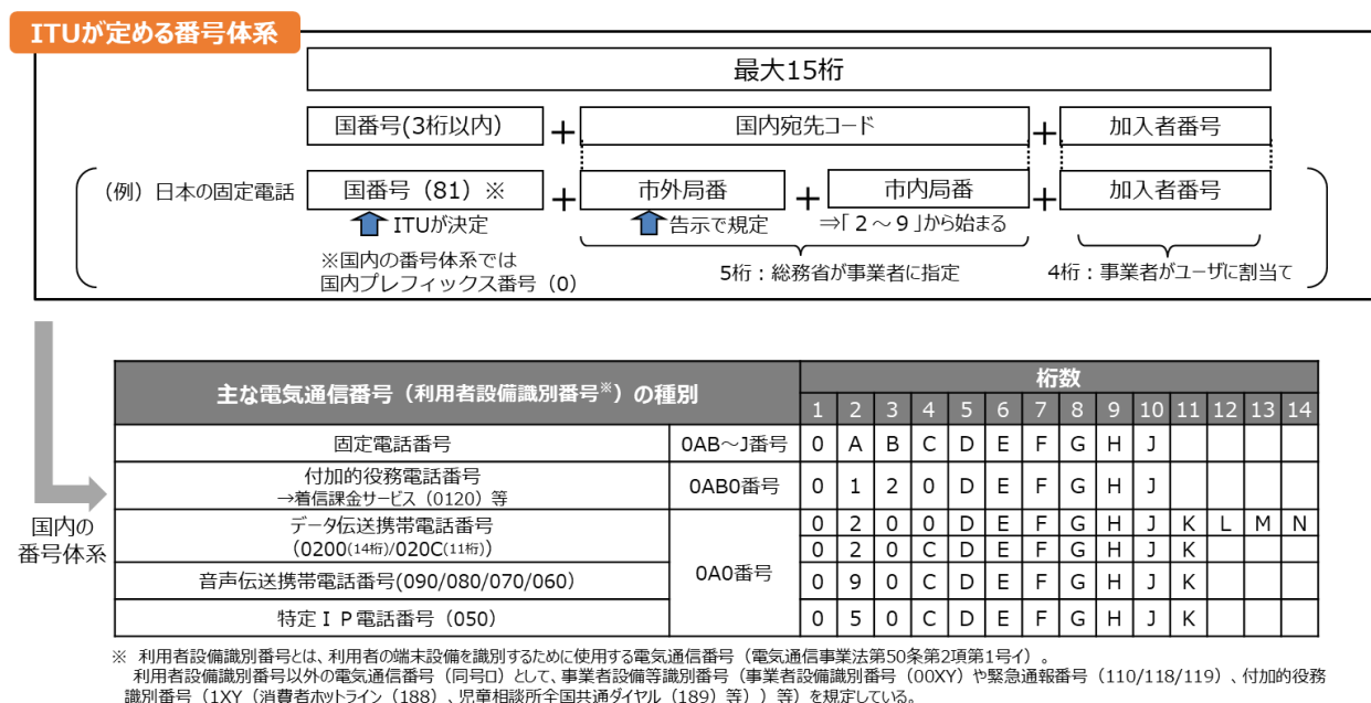
図表 1 電気通信番号の体系
