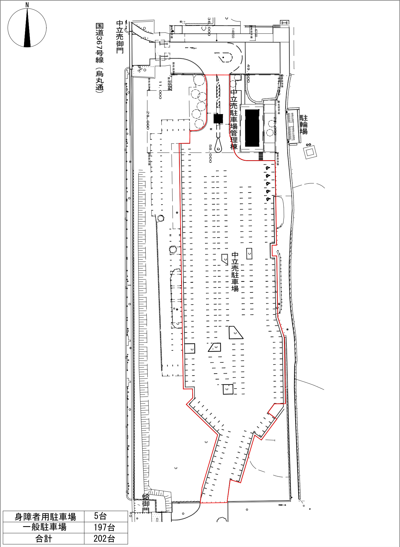
中立的売駐車場配置図平面図
