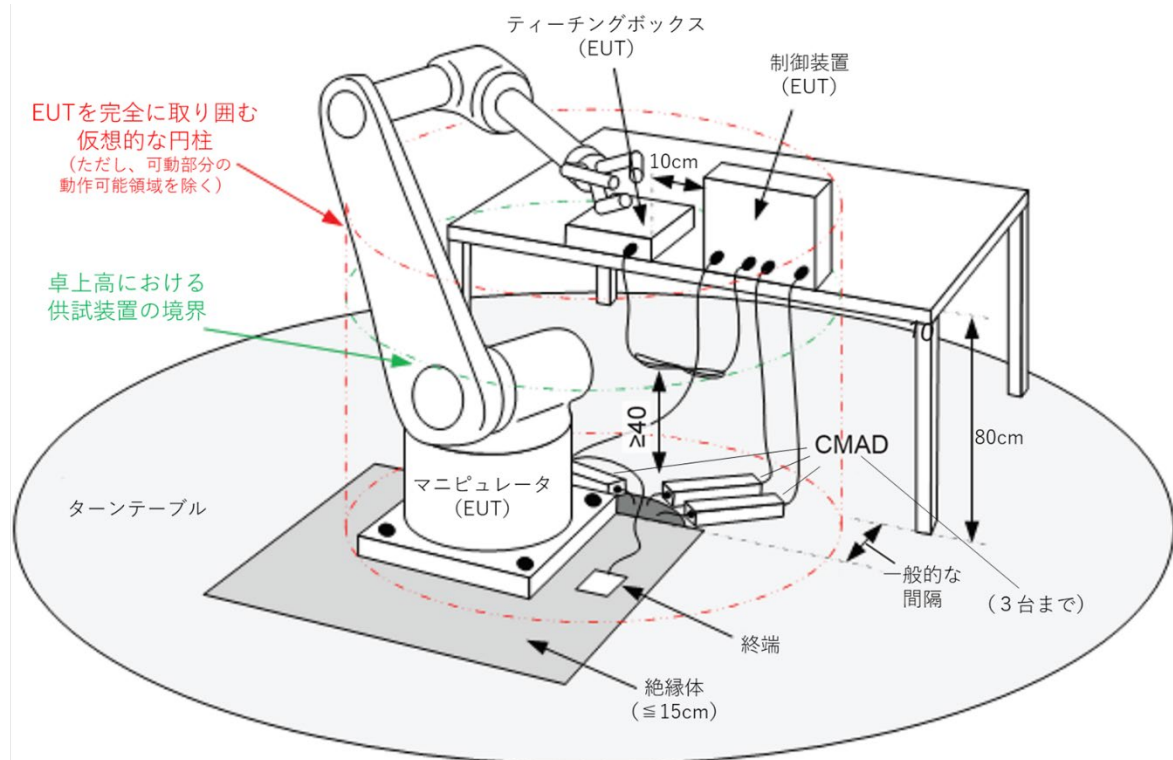
図 9 複合ロボットシステムの放射妨害波測定における一般的配置例
