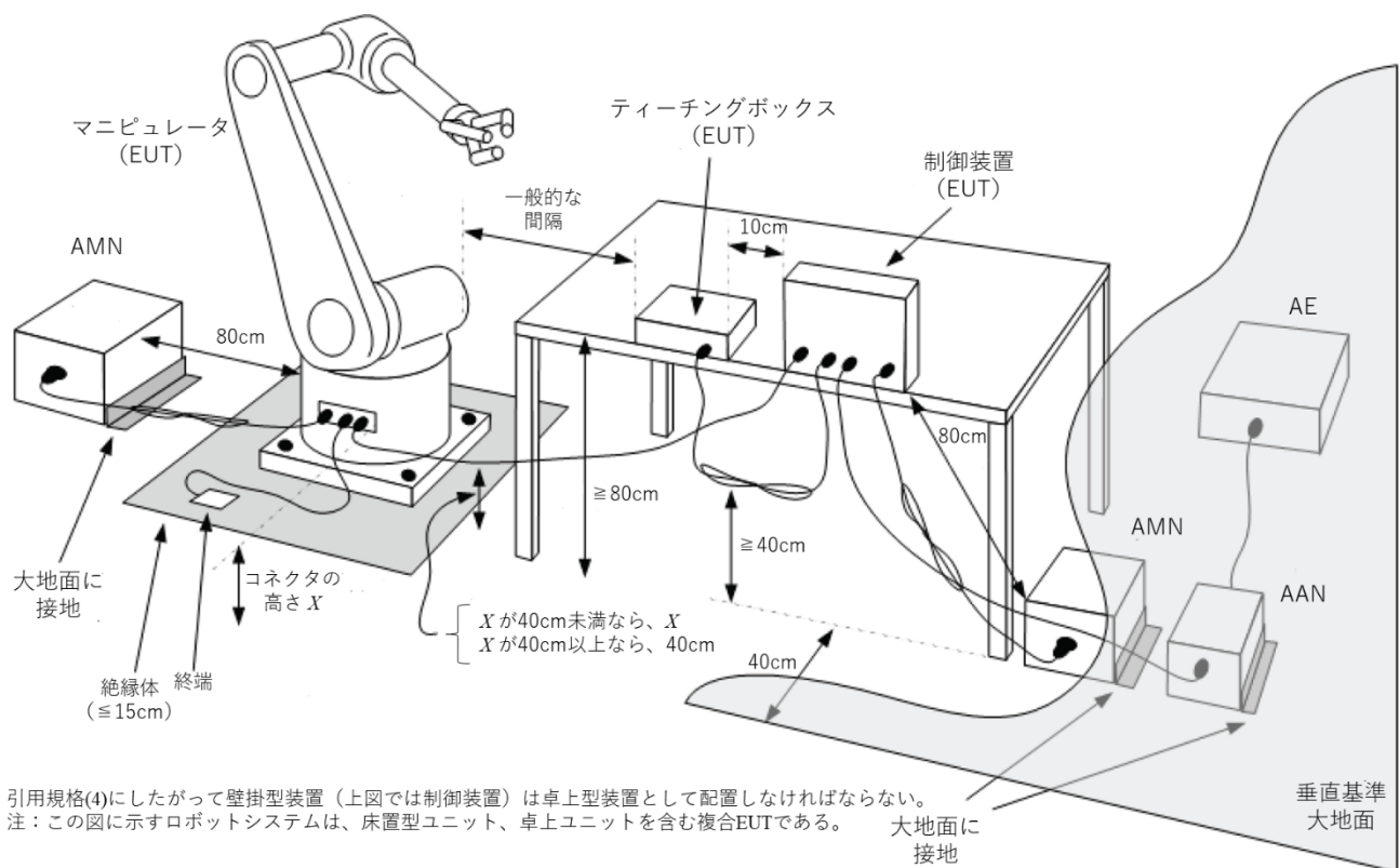
図 8 複合ロボットシステムの伝導妨害波測定における一般的配置例
