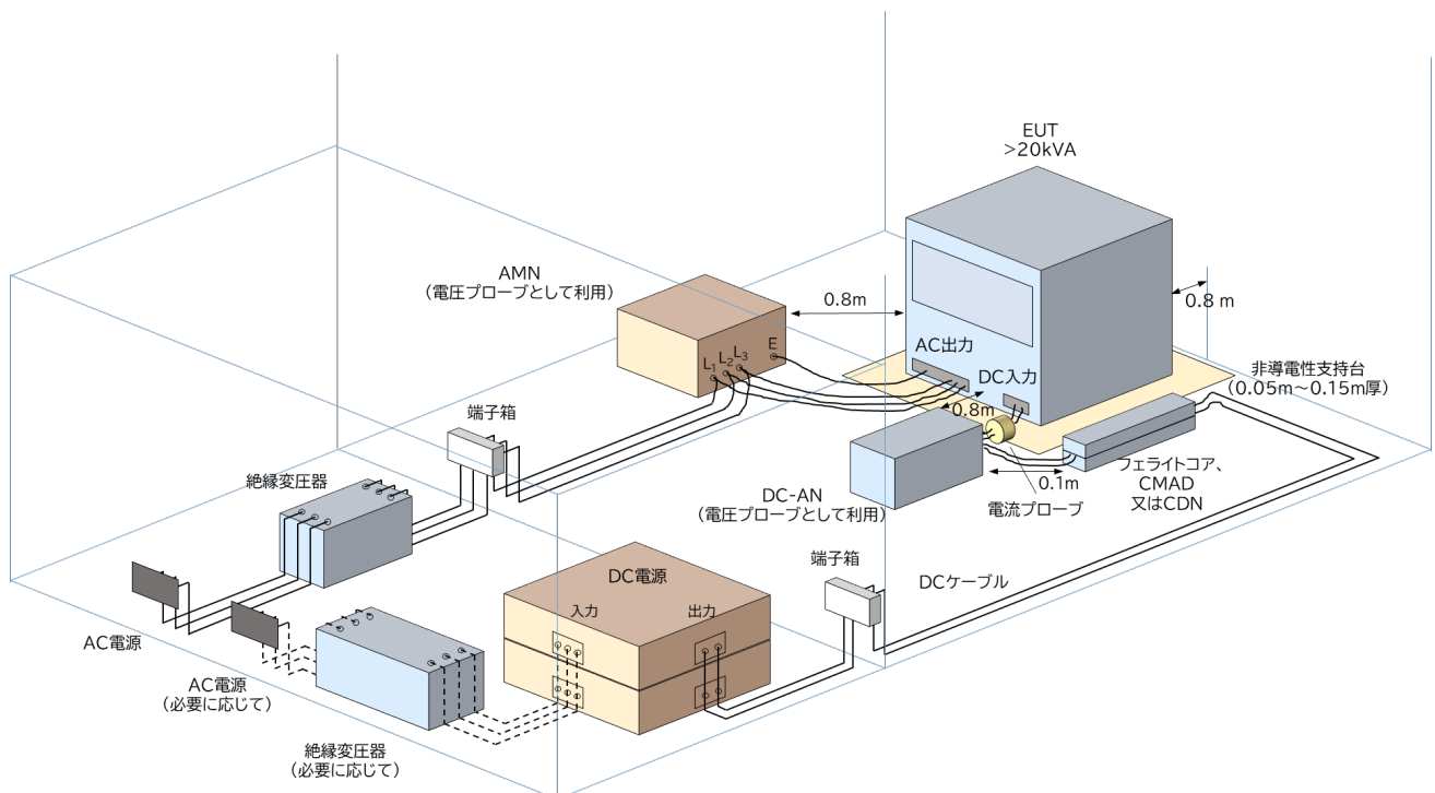
図 14 電圧プローブとして用いる DC-AN と電流プローブを用いる低電圧 DC 電源ポートの伝導妨害波測定の一般的な測定配置（三次元図）
