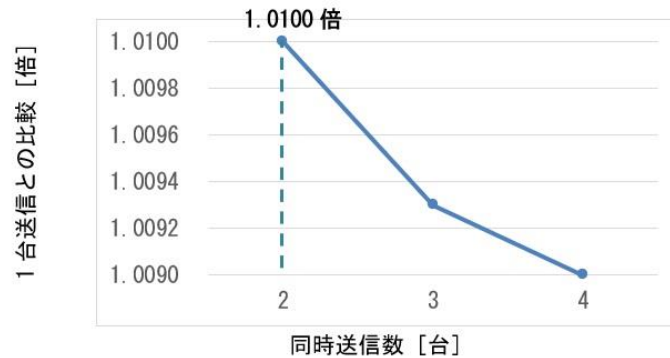
図 56 VHF-IoT の同時送信検討結果（上側帯域、L=1m）
