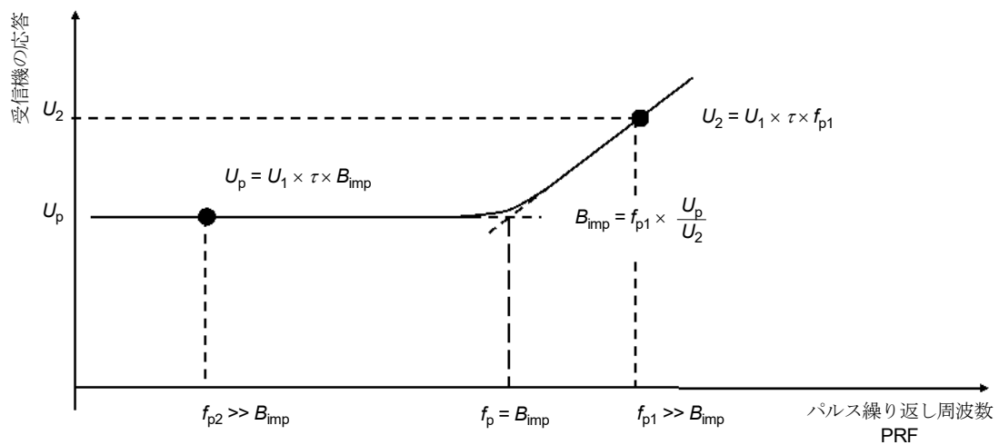
図 E.7 - インパルス帯域幅の計算
