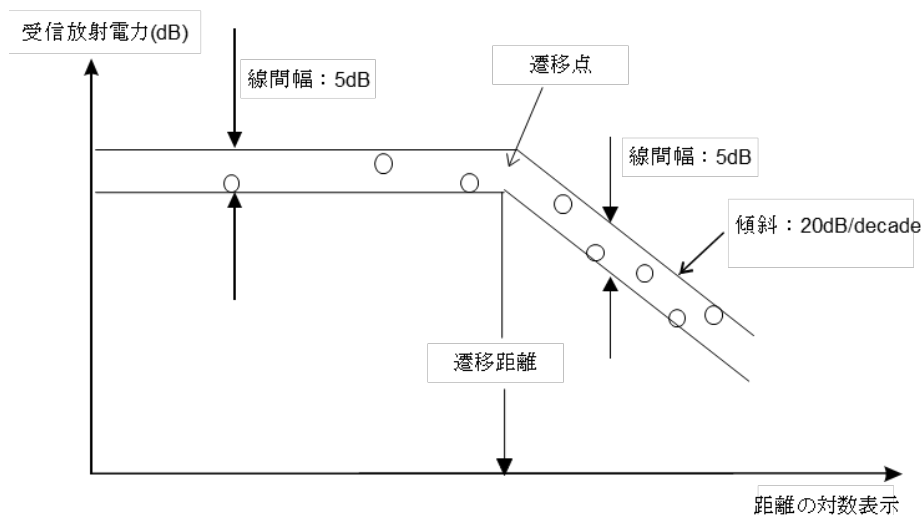
図 22 - 遷移距離の決定
