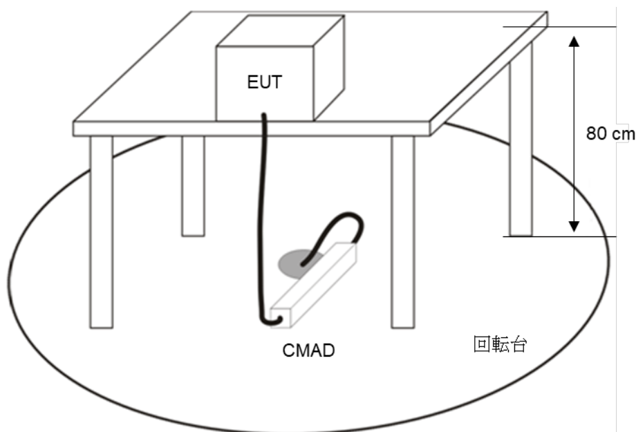
図 11 - OATS 又は SAC における卓上型装置に対する CMAD の配置
