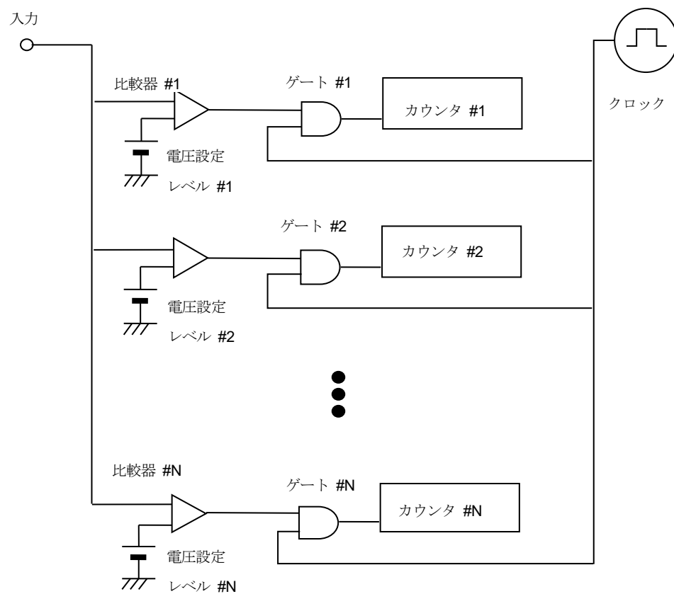
図 G.1 - A/D 変換器を使用しない APD 測定回路のブロック図
