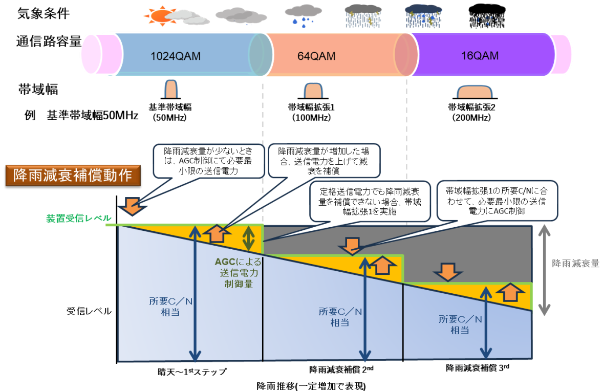
図 2-11 FWA 高度化の装置の降雨減衰補償動作図
