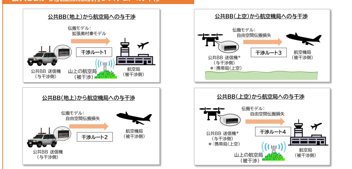
図 24 公共 BB が与干渉の場合の航空無線航行システムとの共用検討モデル
