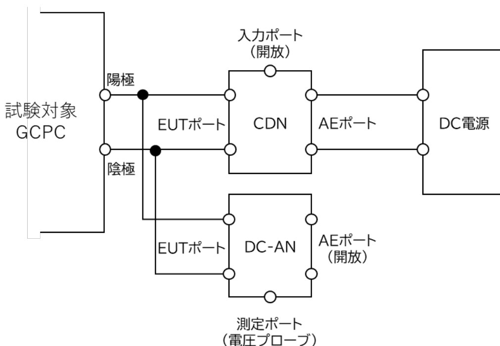
図 12 終端及び電圧プローブとして DC-AN を用いた低電圧 DC 電源ポートの伝導妨害波測定のための一般的な測定配置
